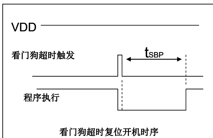
图 19: 看门狗超时溢出时序图
