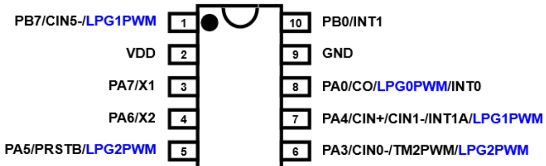
PMS152G-M10 (MSOP10-118mil)
