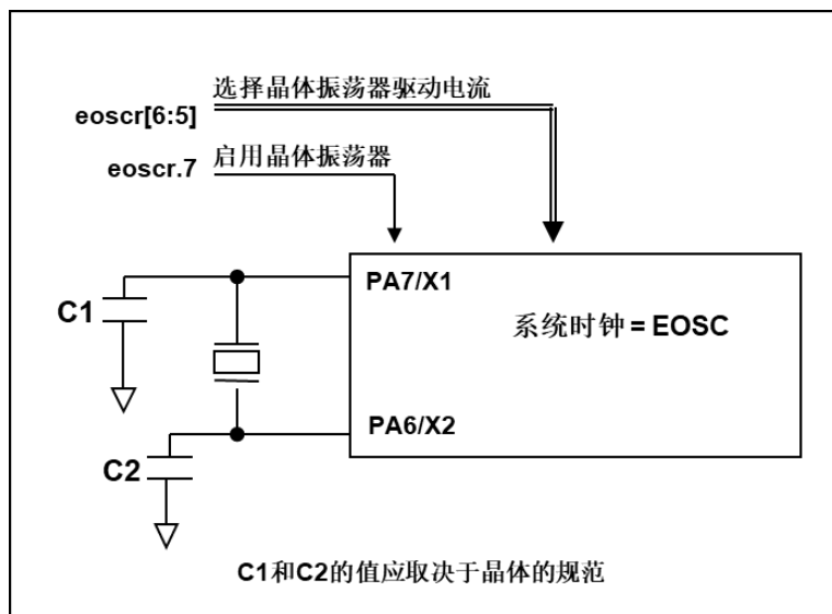
图 2：晶体振荡器的硬件连接图
