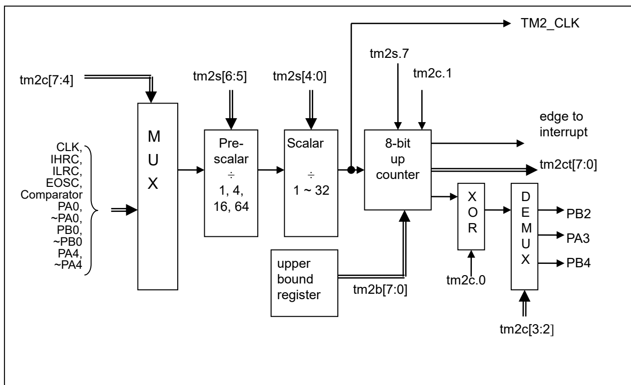
图 10: Timer2 硬件框图
