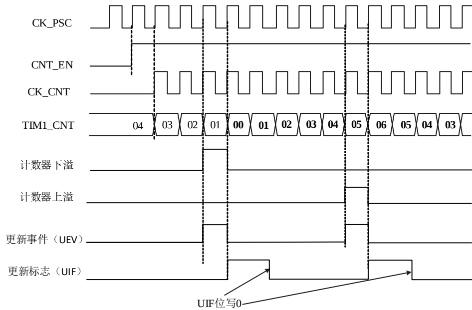
图 13-11 中心对齐模式下配置预分频器为 1 分频上/下溢事件时序图
