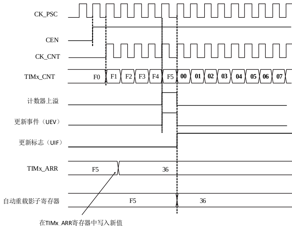
图 14-7 递增计数模式下计数器时序图，ARPE=1 时更新事件
