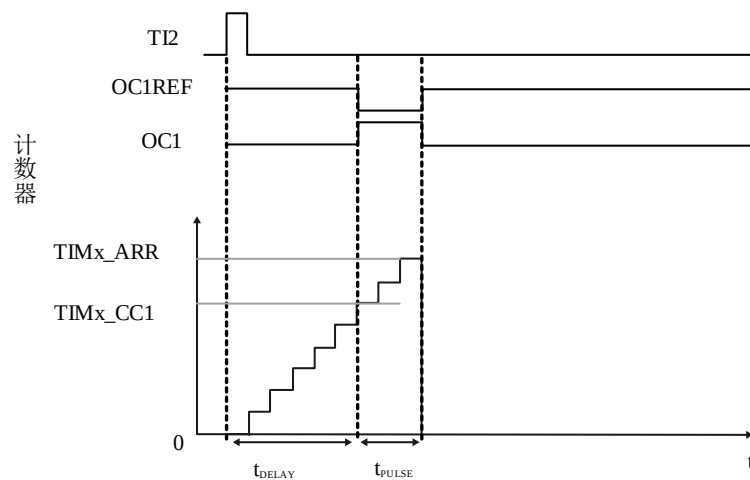
图 14-18 单脉冲模式示例
