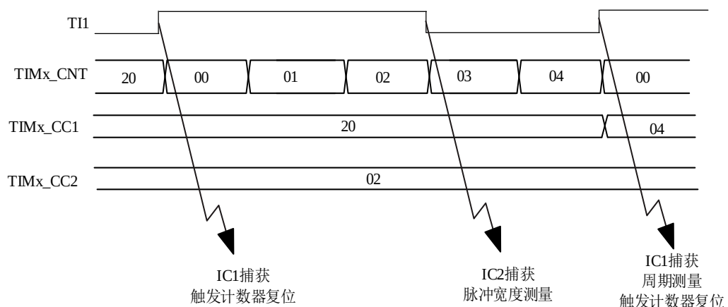
图 14-14 PWM 输入模式的时序
