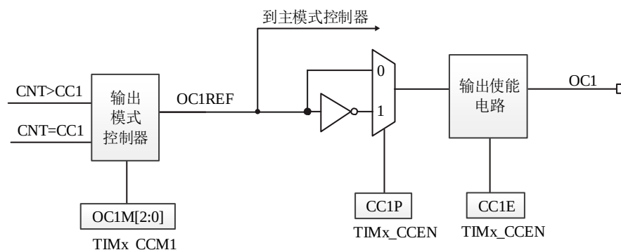
图 14-13 捕获/比较通道的输出连接图（通道 1）
