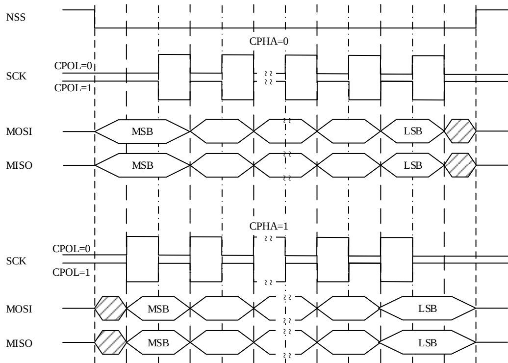
图 21-5 通信模式时序
