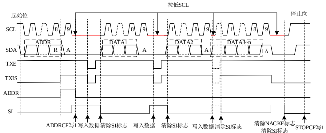
图 19-7 使能时钟低电平延长单字节控制发送数据
