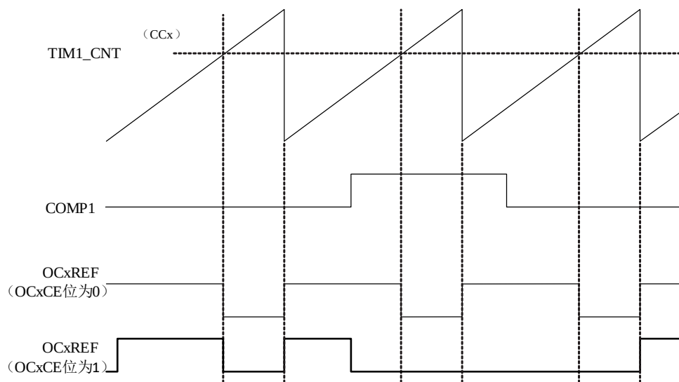
图 13-25 清除 TIM1 的 OCxREF
