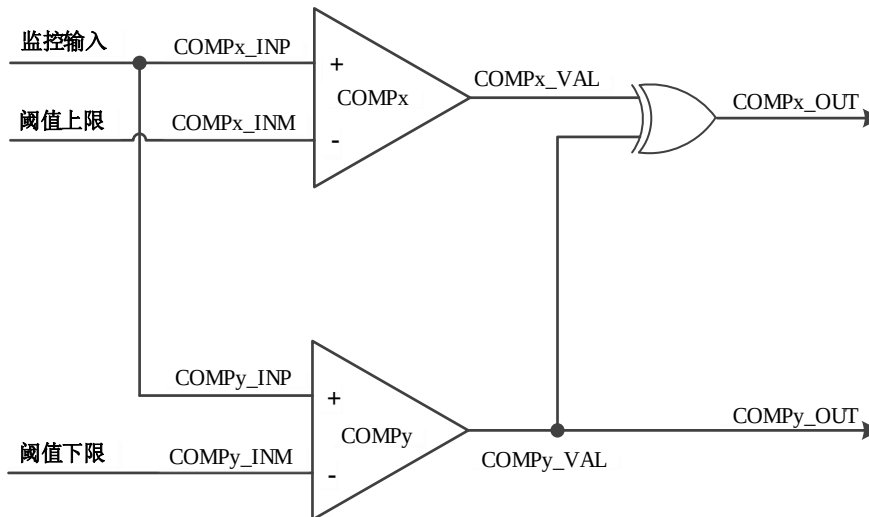
图 12-2 窗口比较器结构 (1)
