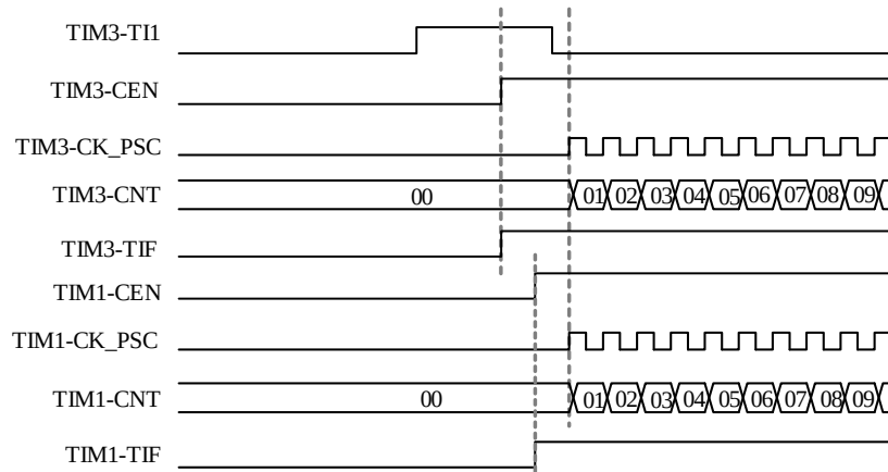
图 14-25 使用 TIM3 的 TI1 输入触发 TIM3 和 TIM1
