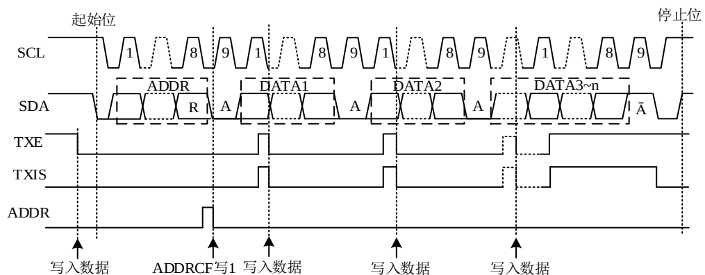
图 19-9 禁止时钟低电平延长发送数据
