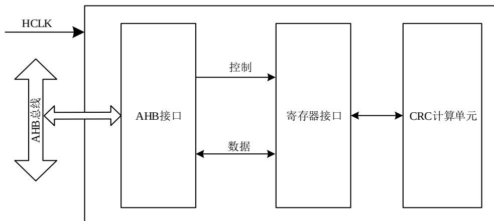
图 10-1 CRC 框图
