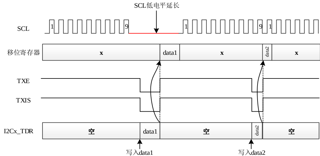
图 19-6 多字节控制数据发送
