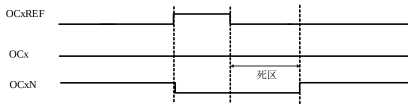
图 13-30 死区时间大于正脉冲宽度的死区波形
