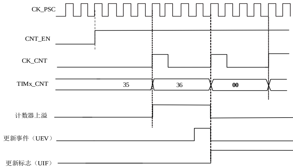
图 14-5 递增计数模式下配置预分频器为 4 分频上溢事件时序图
