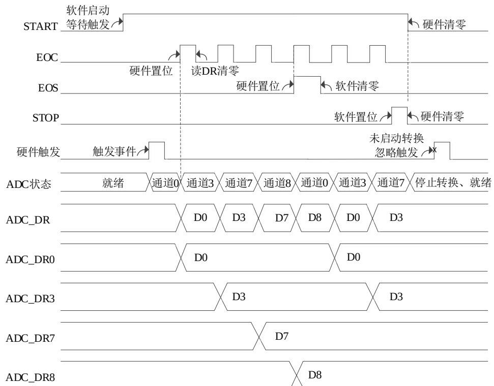
图 11-8 循环扫描转换模式，硬件触发
