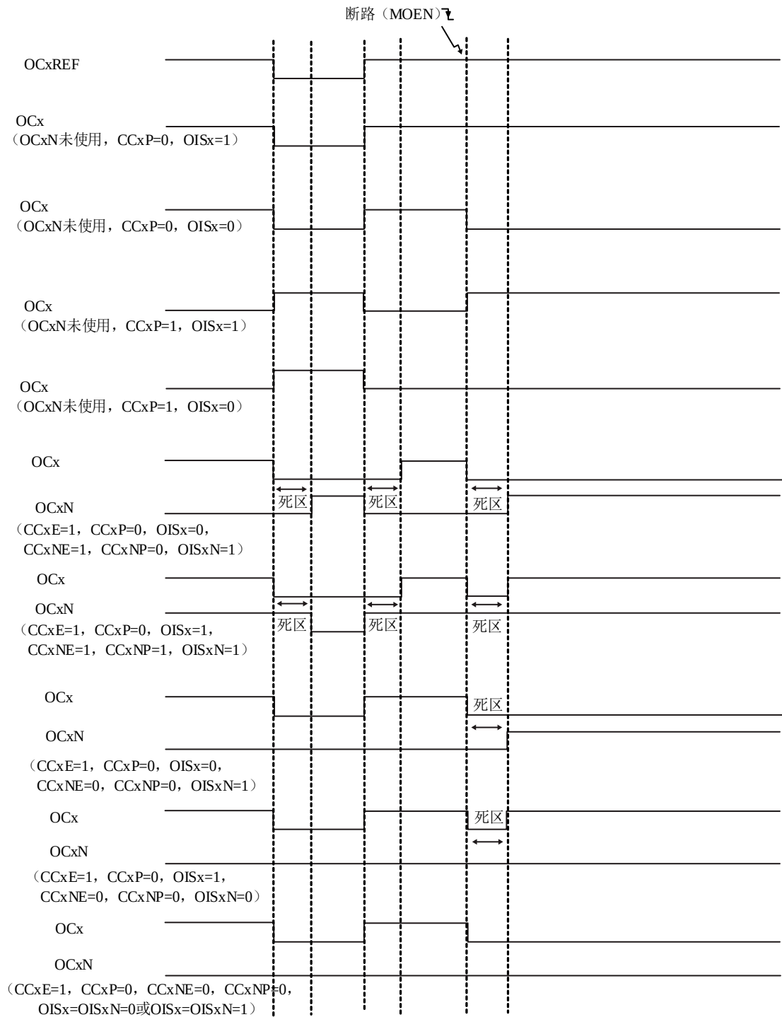
图 13-32 BRK 上断路事件的输出状态（OSSI 位为 1）
