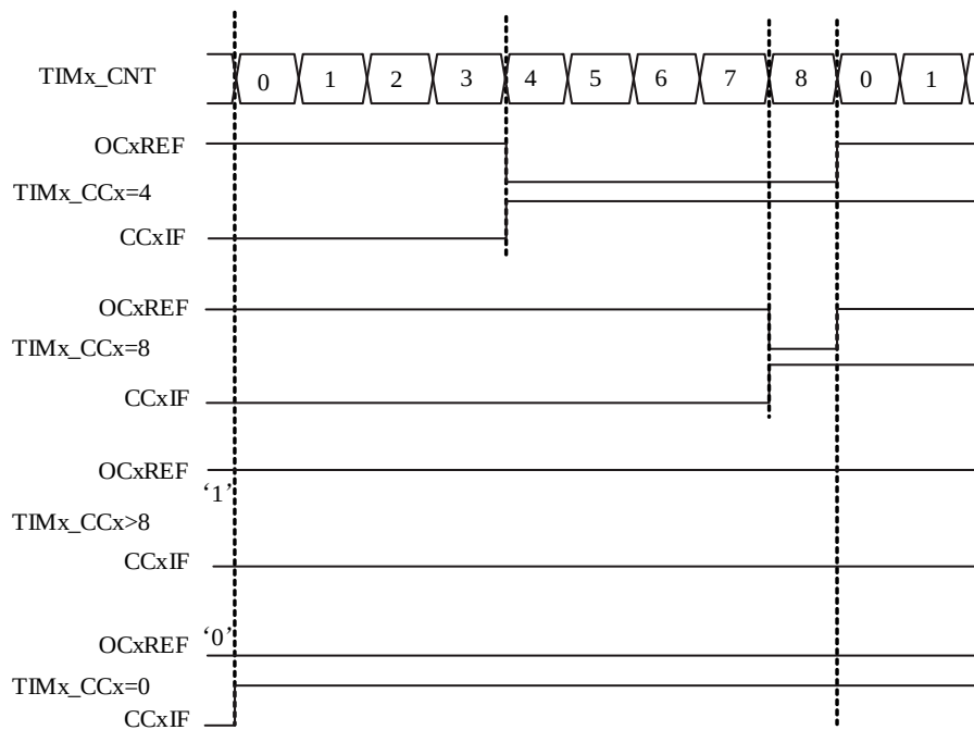
图 14-16 PWM 波形 (TIMx_ARR 寄存器为 8)
