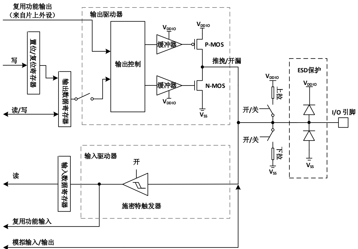
图 7-4 I/O 引脚复用功能配置
