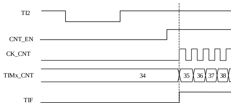
图 14-22 触发模式下的控制时序
