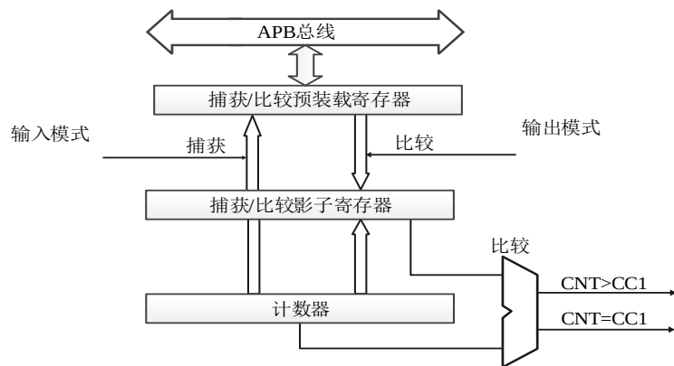
图 14-11 捕获/比较通道
