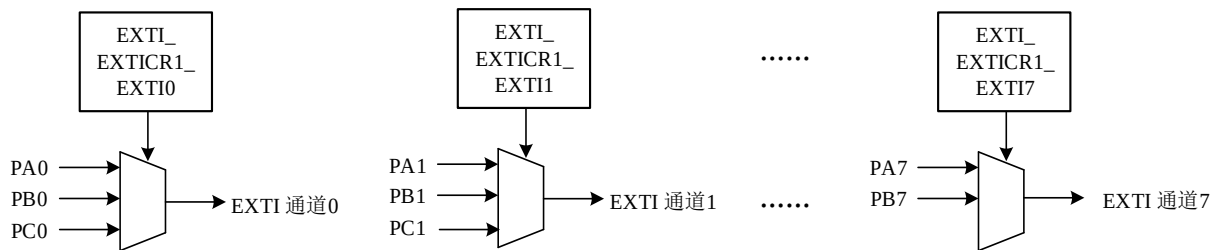
图 9-4 EXTI 多路复用器
