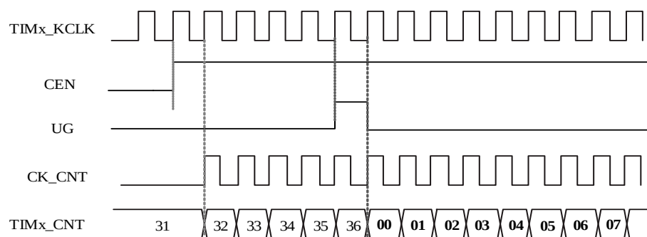
图 14-8 选择内部时钟源时的计数时序图
