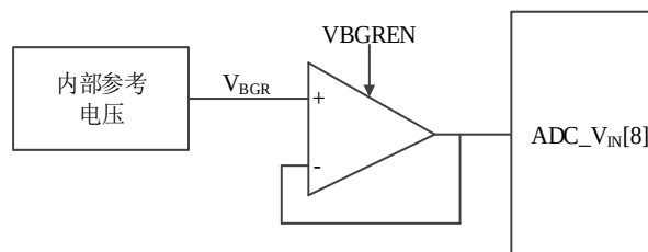
图 11-11 V_{BGR} 输入通道结构
