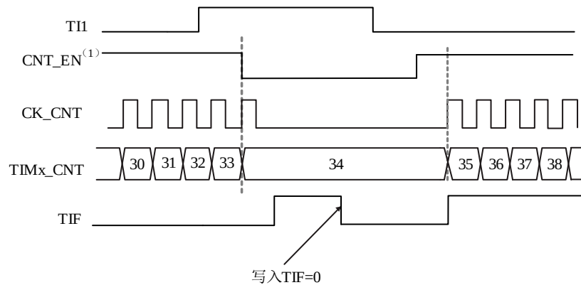
图 14-21 门控模式下的控制时序
