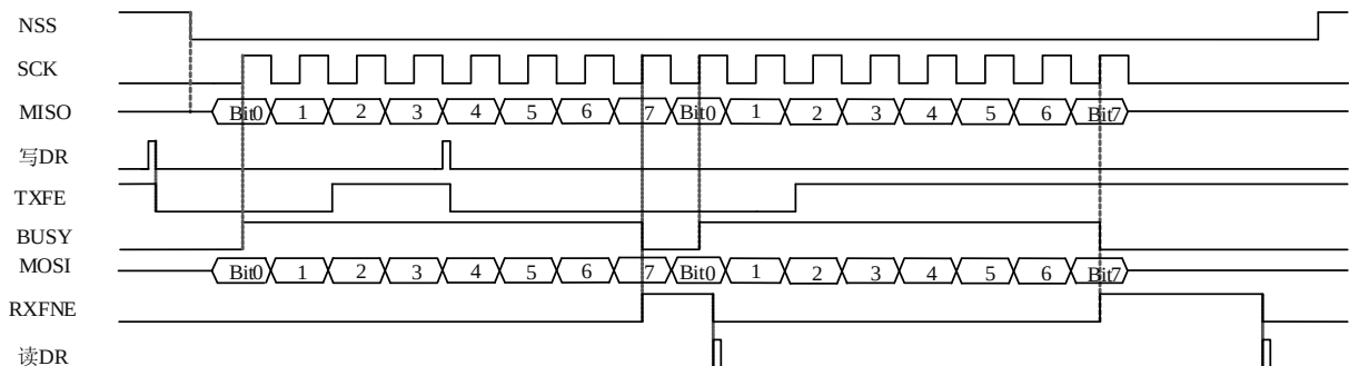
图 21-8 从模式通信时序
