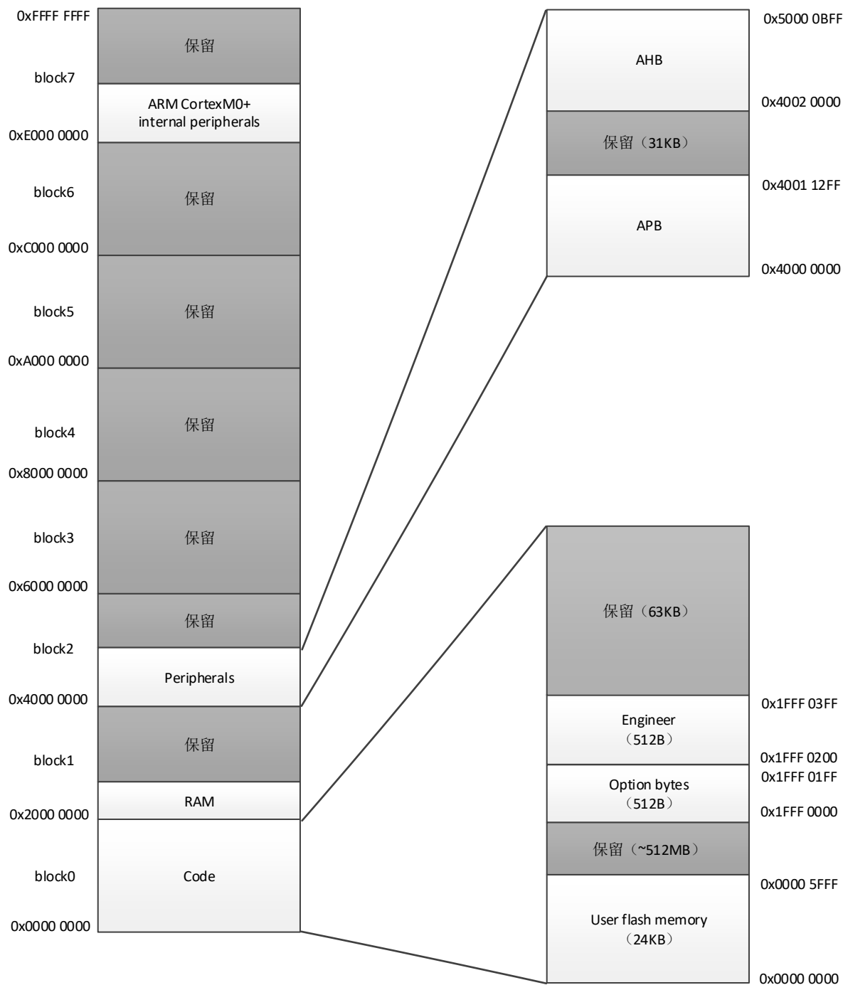
图 3-2 存储器映射
