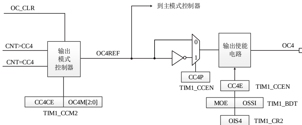
图 13-20 比较通道的输出连接图（通道 4）
