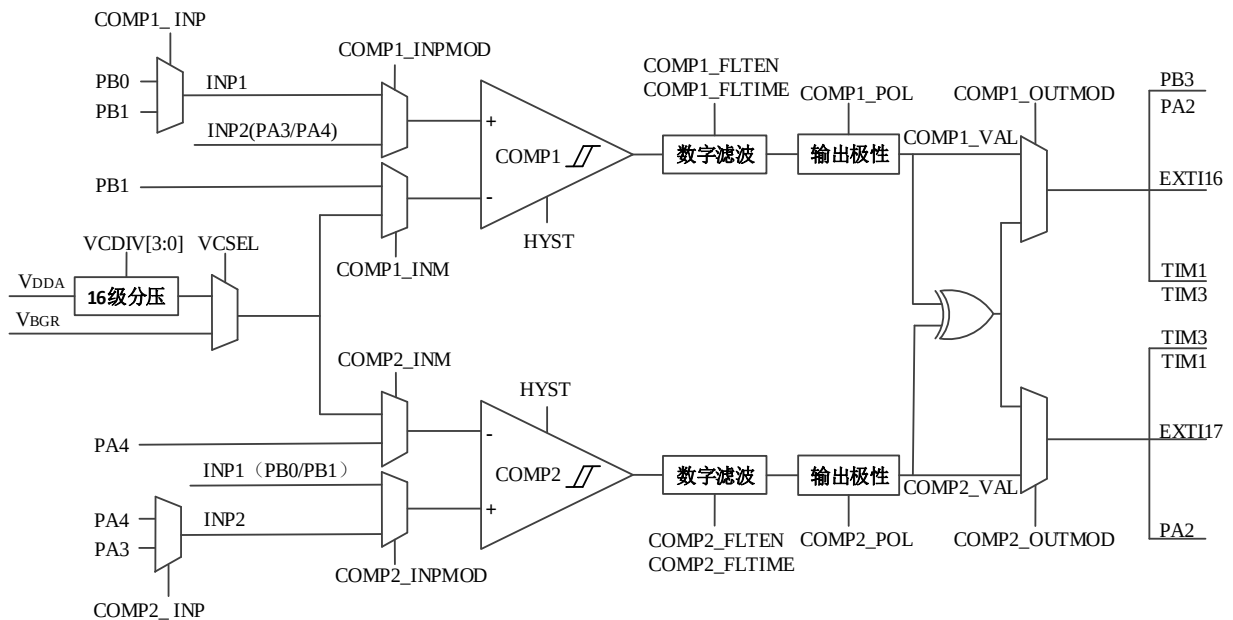
图 12-1 COMP 结构框图
