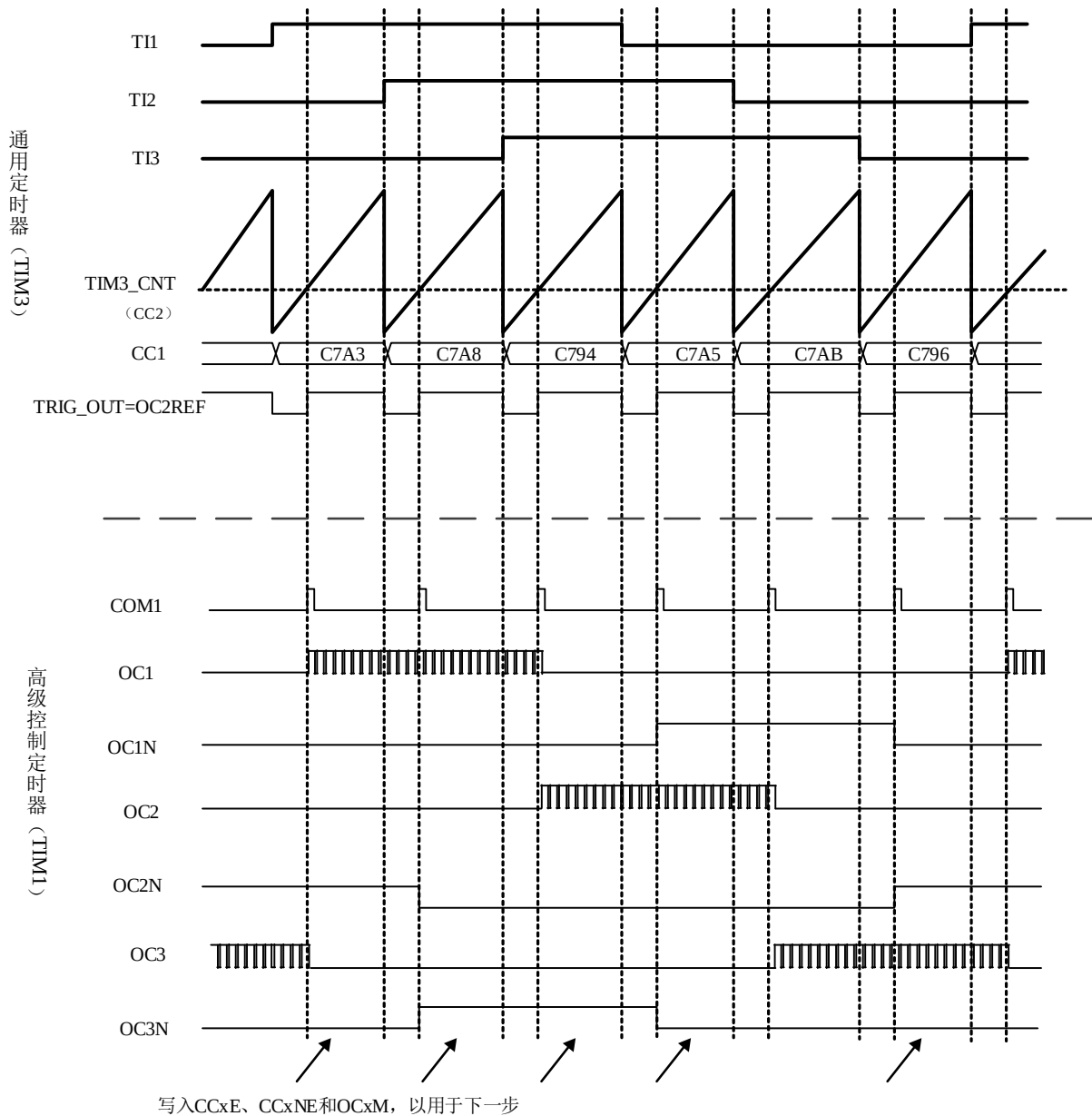
图 13-35 霍尔传感器接口的示例
