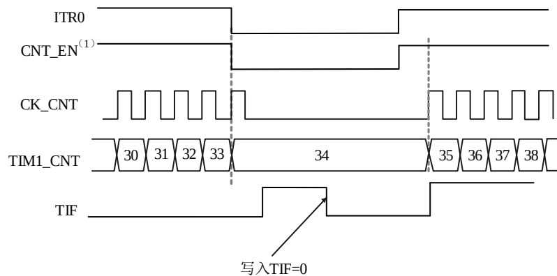
图 13-37 门控模式下的控制时序
