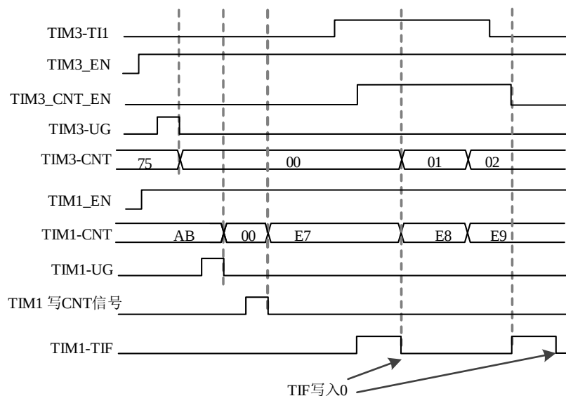
图 14-26 使用 TIM3 的门控信号对 TIM1 实施门控控制
