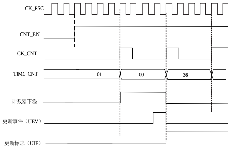
图 13-9 递减计数模式下配置预分频器为 4 分频下溢事件时序图
