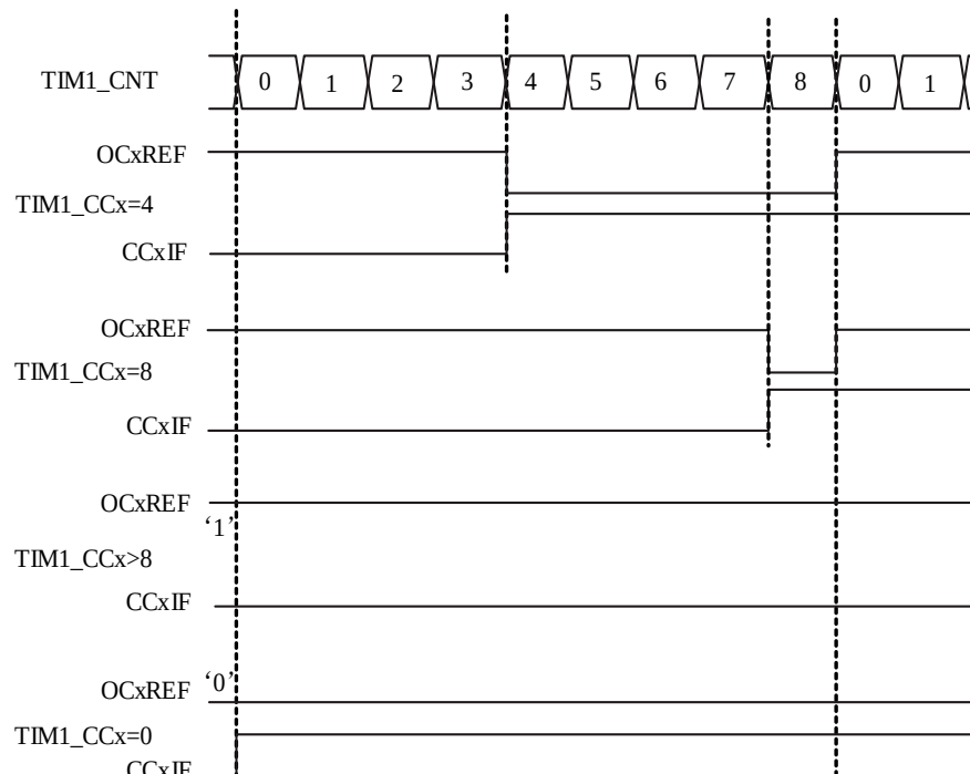
图 13-22 递增计数下的边沿对齐模式 PWM 波形（TIM1_ARR 寄存器为 8）
