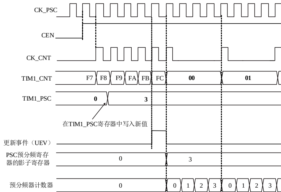
图 13-3 预分频器分频系数由 1 变为 4 时的计数器时序图
