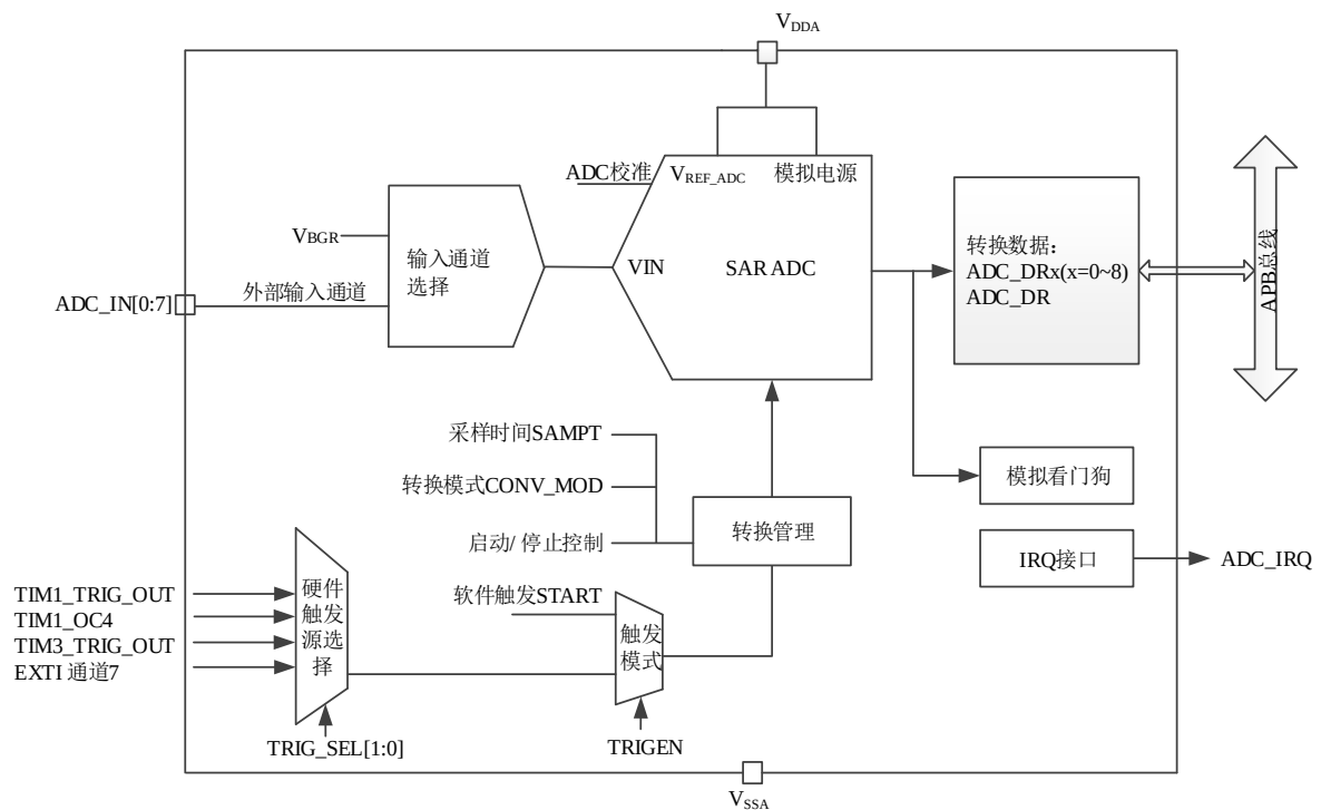
图 11-1 ADC 结构框图
