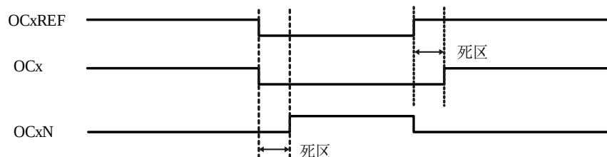
图 13-28 带死区插入的互补输出
