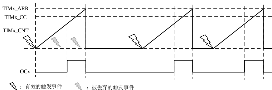
图 14-17 单脉冲输出波形
