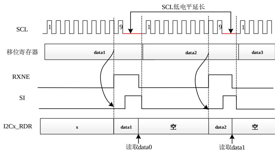
图 19-3 单字节控制数据接收
