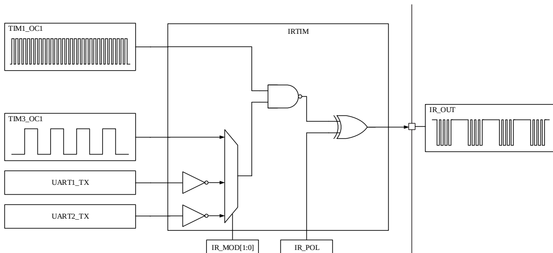
图 16-1 IRTIM 框图
