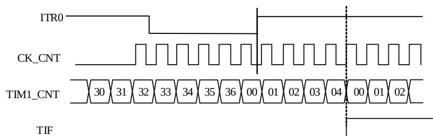
图 13-36 复位模式下的控制时序
