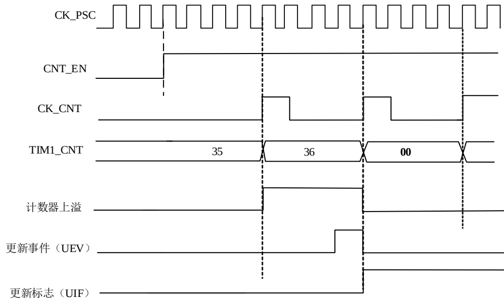
图 13-5 递增计数模式下配置预分频器为 4 分频上溢事件时序图
