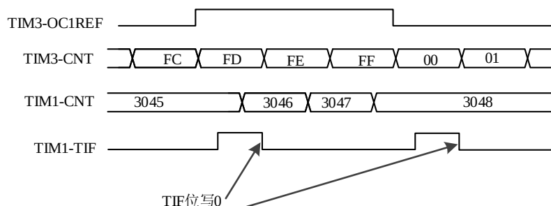
图 14-24 使用 TIM3 的 OC1REF 信号对 TIM1 实施门控控制
