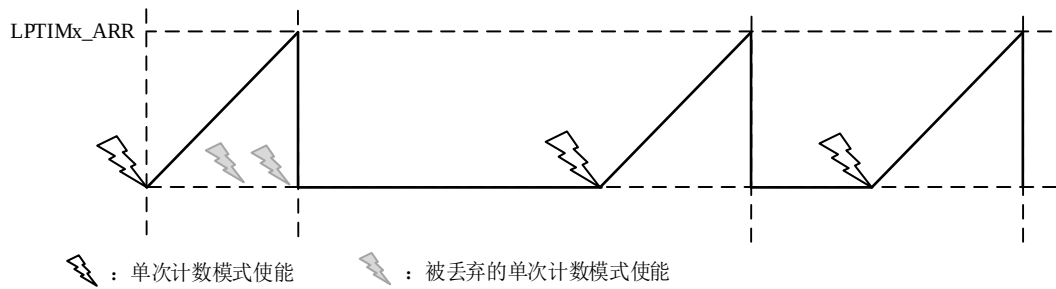
图 15-2 单次计数模式使能说明
