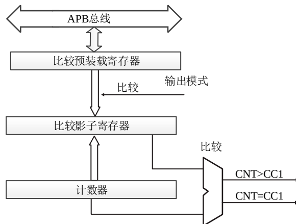
图 13-18 比较通道
