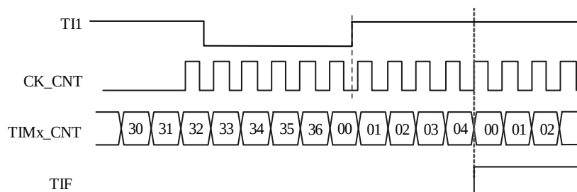
图 14-20 复位模式下的控制时序
