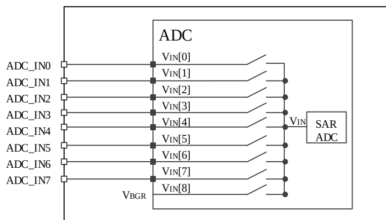
图 11-2 ADC 输入通道
