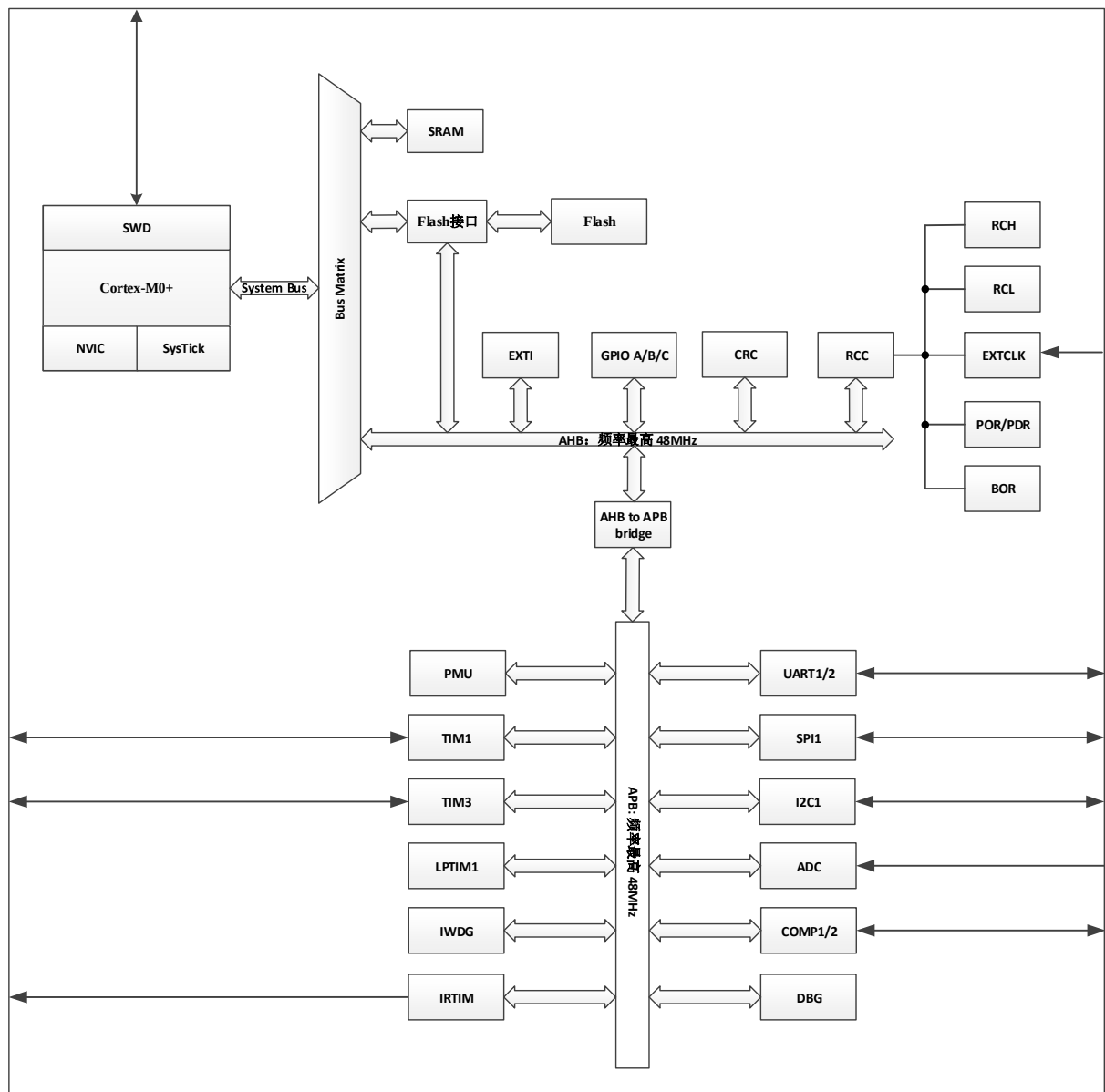
图 3-1 系统架构示意图
