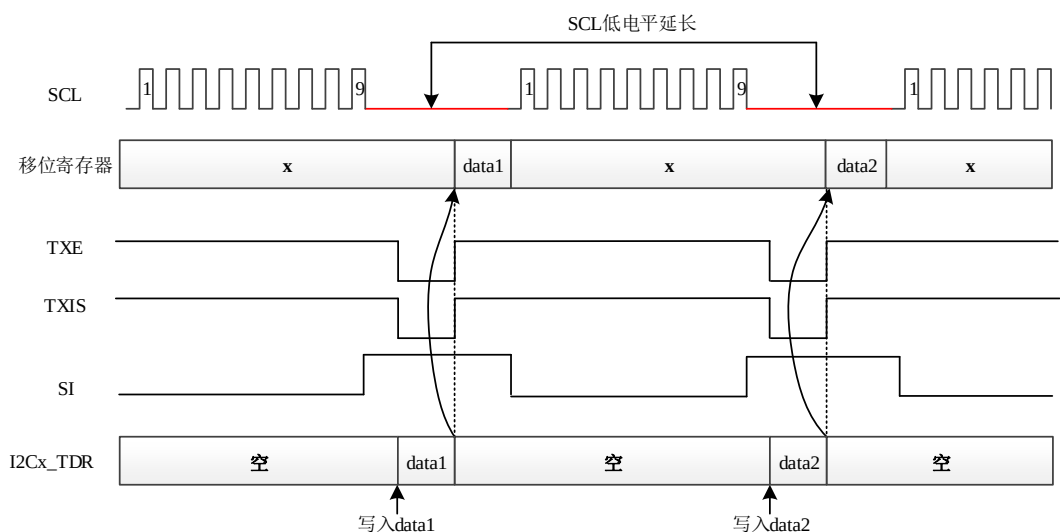
图 19-5 单字节控制数据发送
