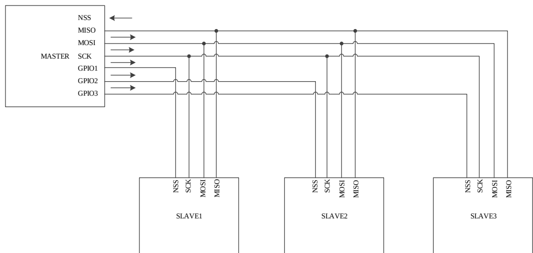
图 21-3 单主多从应用
