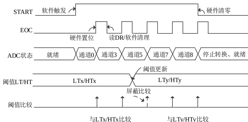
图 11-10 模拟看门狗阈值更新 (1)
