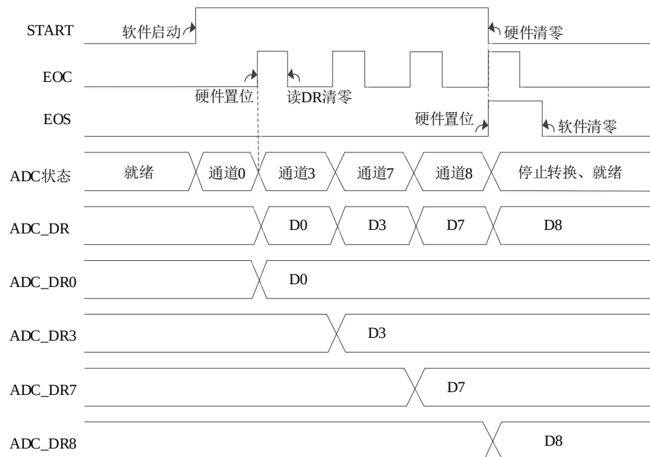
图 11-5 单次扫描转换模式，软件触发
