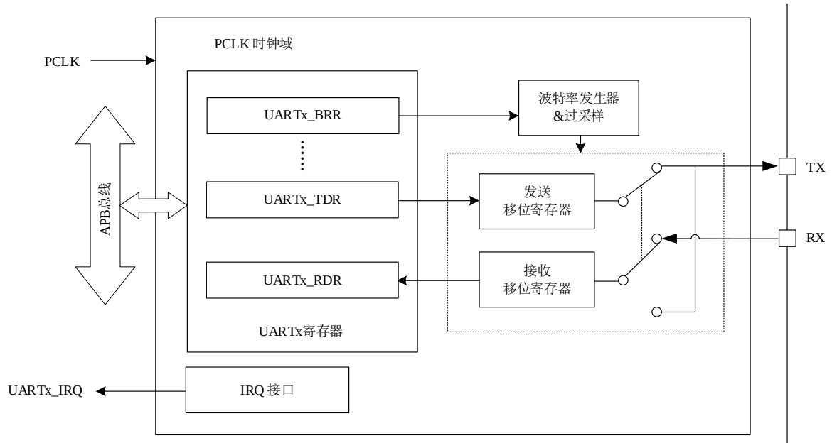
图 20-1 UARTx 框图 (x=1、2)
