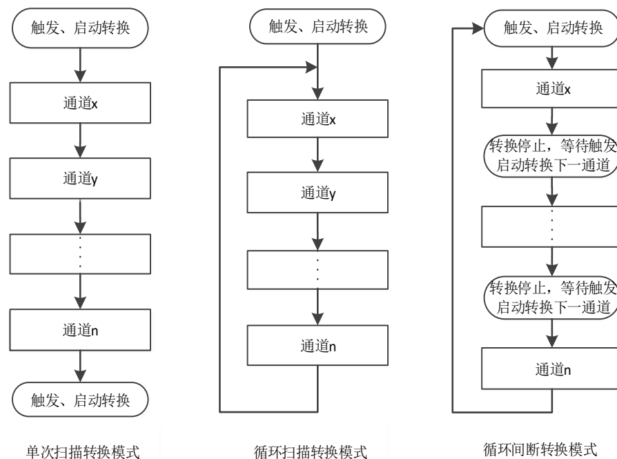
图 11-3 ADC 转换模式
