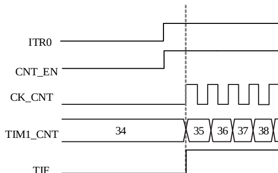
图 13-38 触发模式下的控制时序
