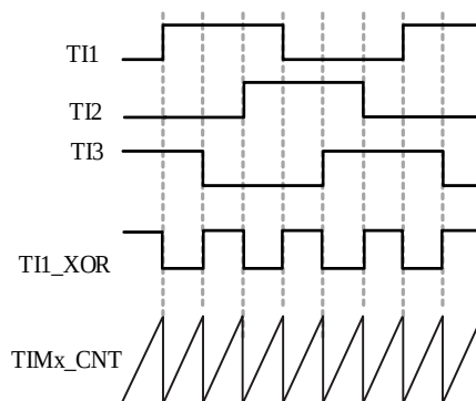
图 14-19 测量 3 个信号边沿之间的时间间隔
