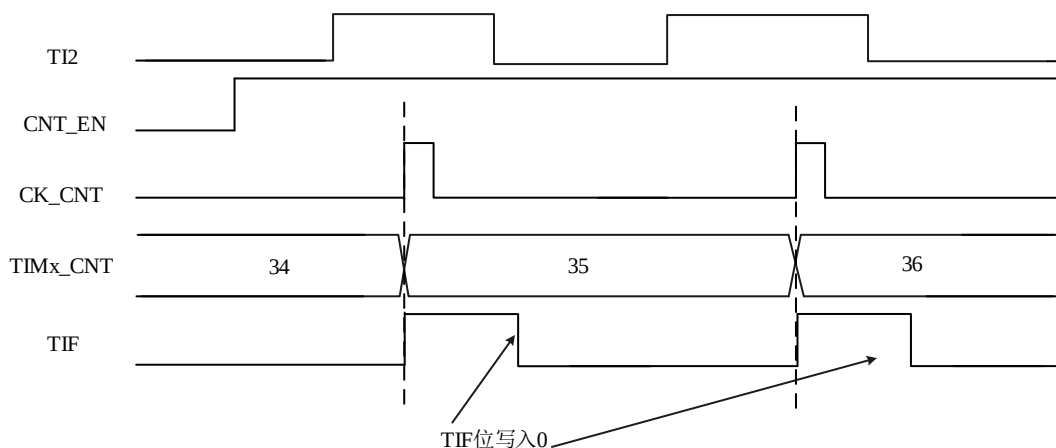
图 14-10 选择时钟模式 1 时的时序图
