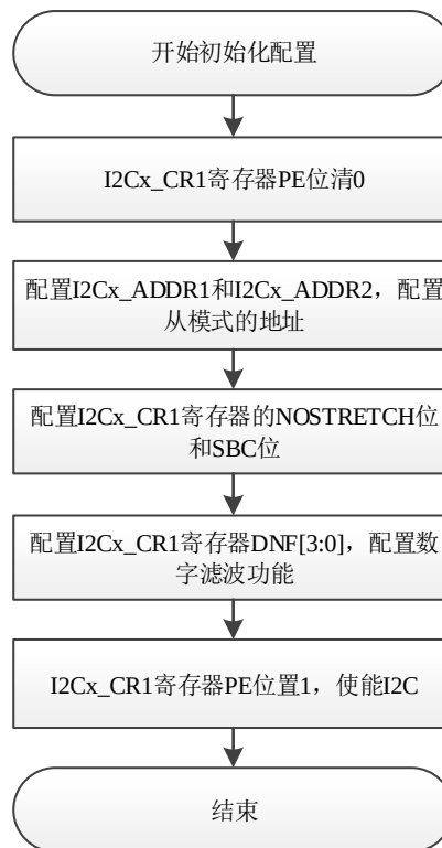
图 19-2 I2C 初始化流程
