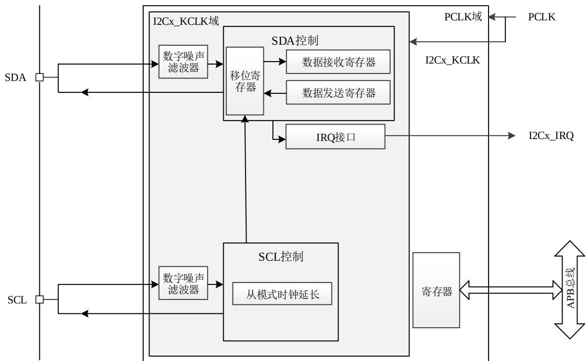
图 19-1 I2Cx 框图 (x=1)
