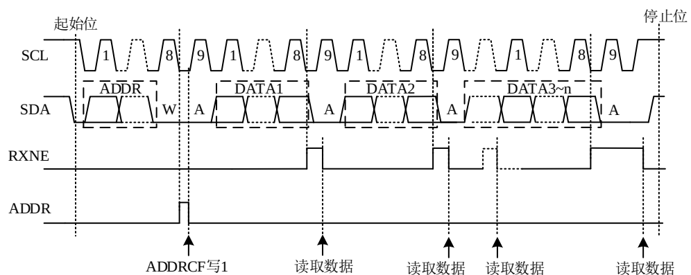
图 19-12 禁止时钟低电平延长接收数据
