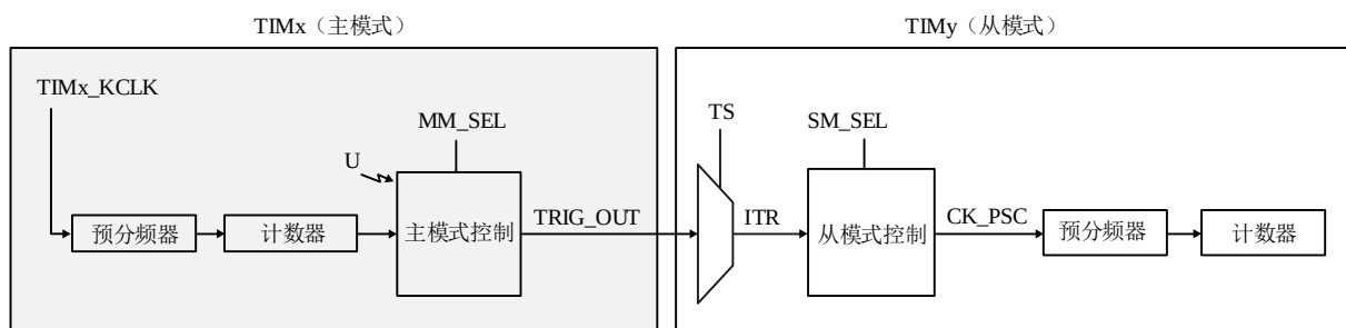
图 14-23 主从定时器连接示例图
