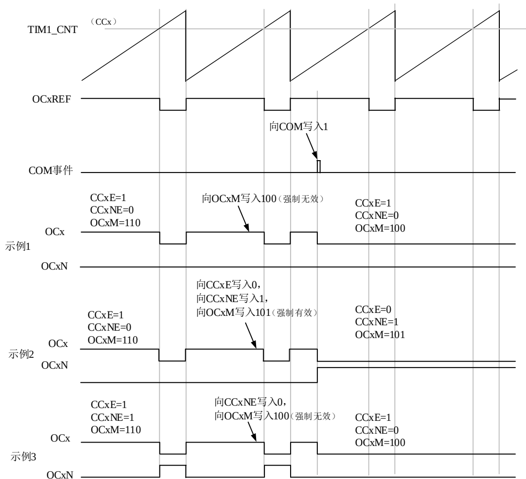
图 13-34 COM 事件生成 6 步 PWM 的示例 (OSSR=1)
