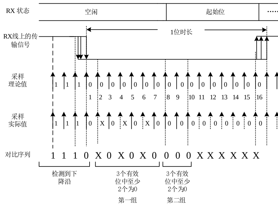
图 20-5 起始位检测
