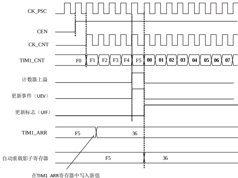
图 13-7 递增计数模式下计数器时序图，ARPE=1 时更新事件
