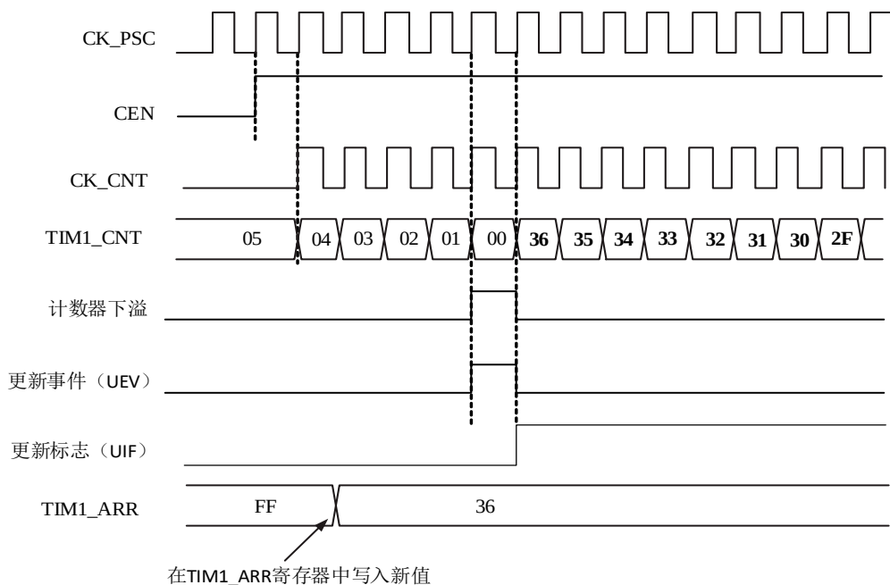
图 13-10 递减计数模式下计数器时序图，ARPE=0 时更新事件
