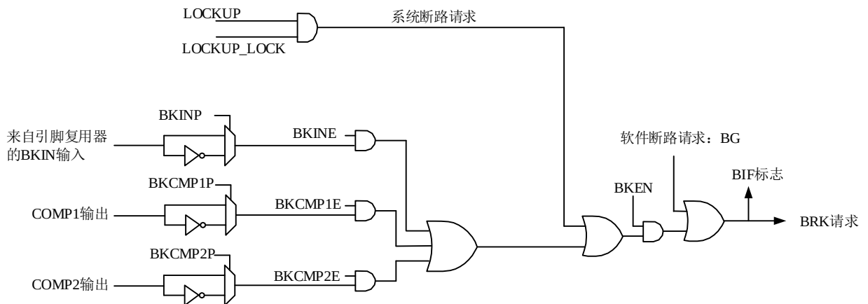
图 13-31 断路电路概述
