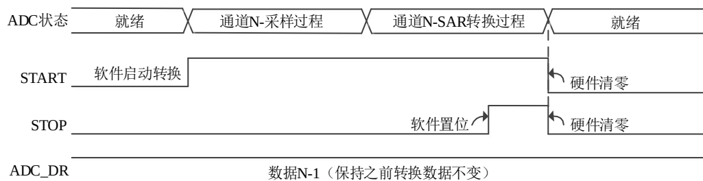
图 11-4 停止正在进行的转换
