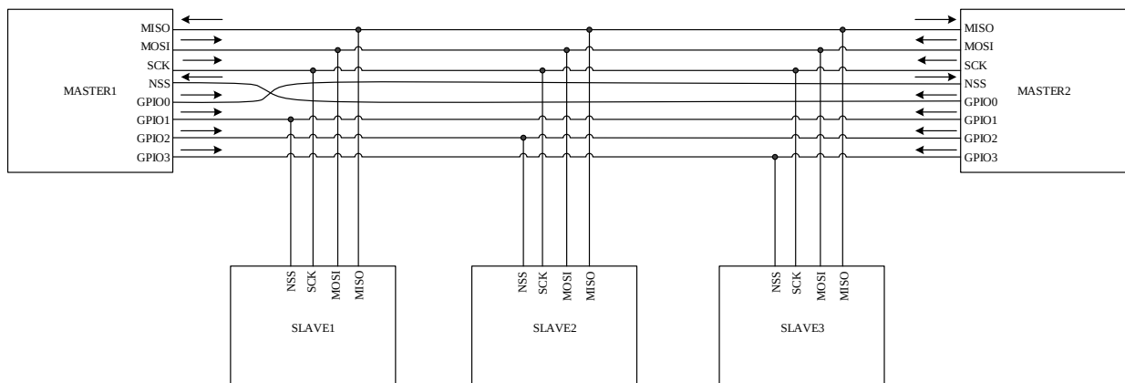
图 21-4 多主多从应用
