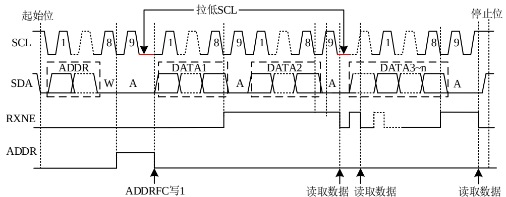
图 19-11 使能时钟低电平延长多字节控制接收数据
