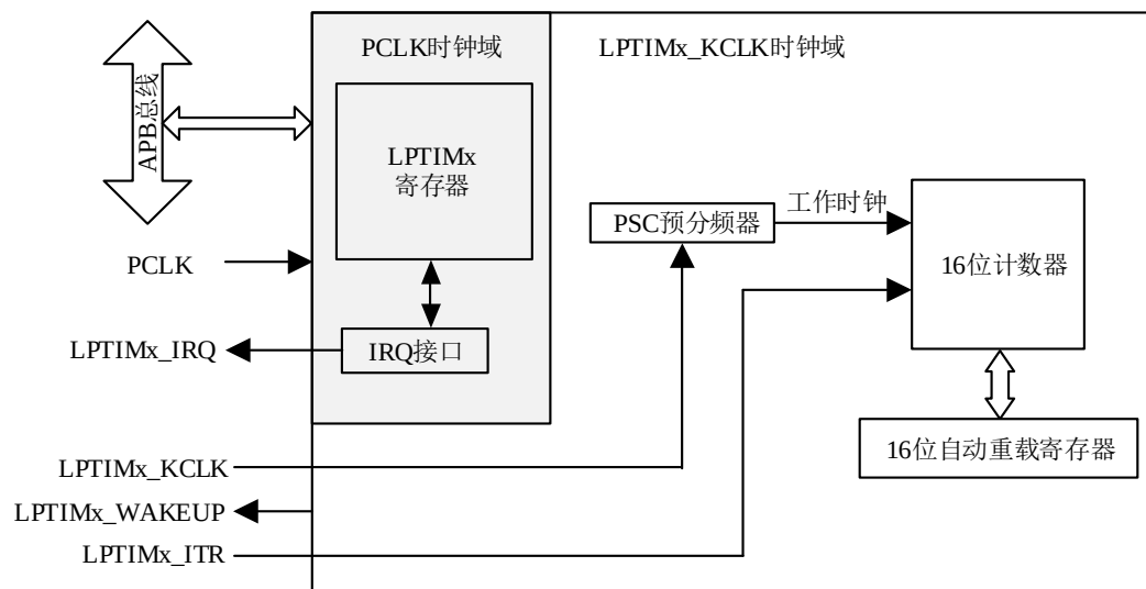
图 15-1 LPTIM x 框图 (x=1)
