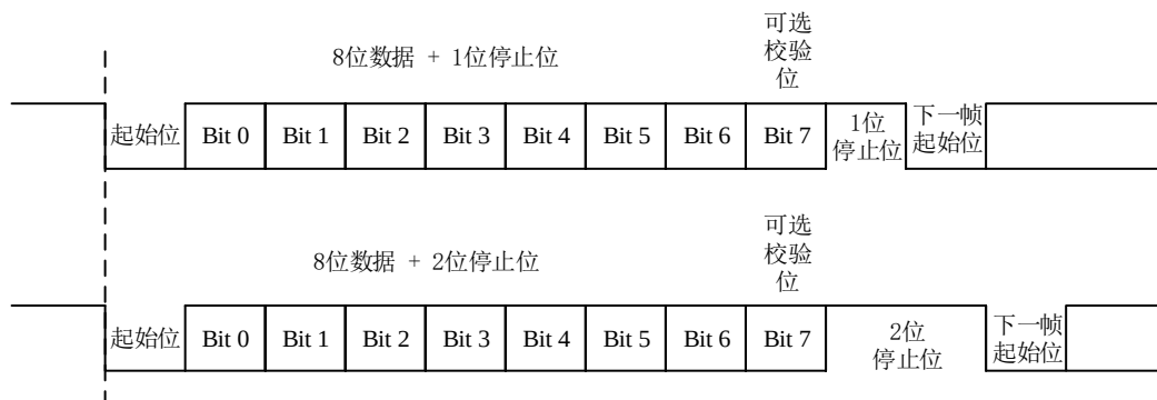
图 20-3 可编程停止位示例
