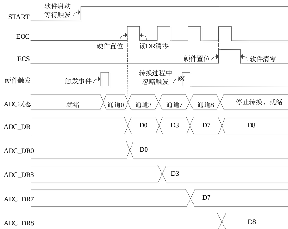
图 11-7 单次扫描转换模式，硬件触发
