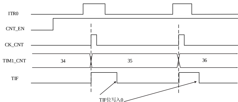
图 13-17 选择时钟模式 1 时的时序图
