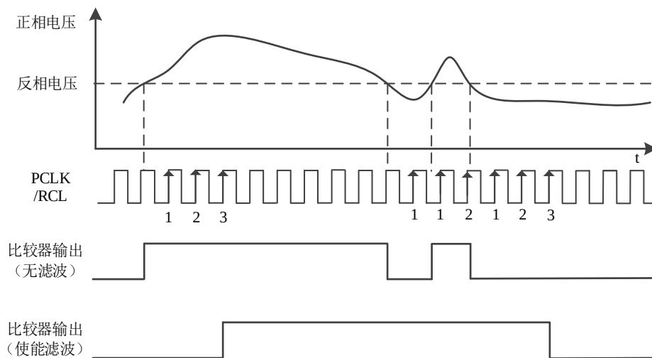
图 12-3 COMP 输出滤波 (1)
