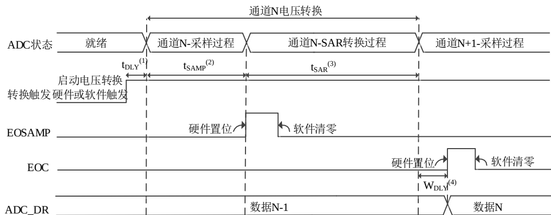
图 11-9 ADC 转换时序
