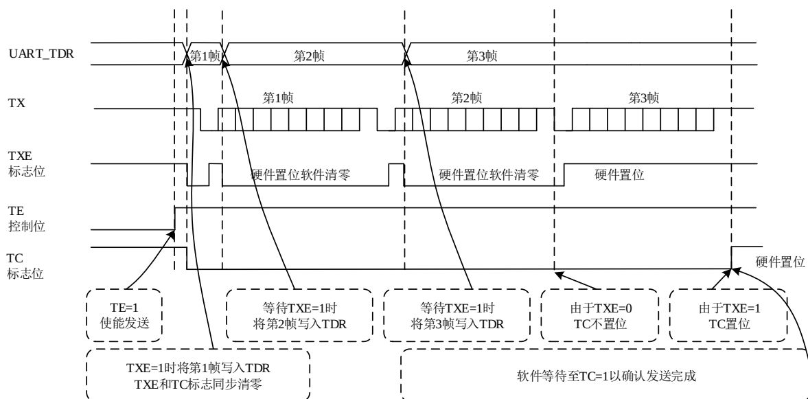
图 20-4 发送过程 TC 和 TXE 的动作
