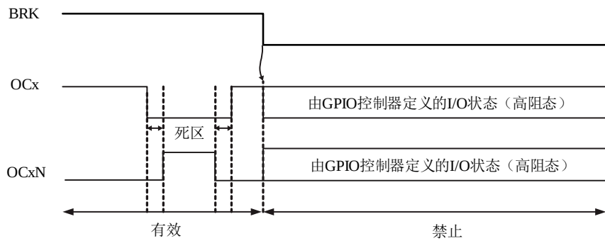
图 13-33 BRK 使能后的 PWM 输出状态 (OSSI=0)
