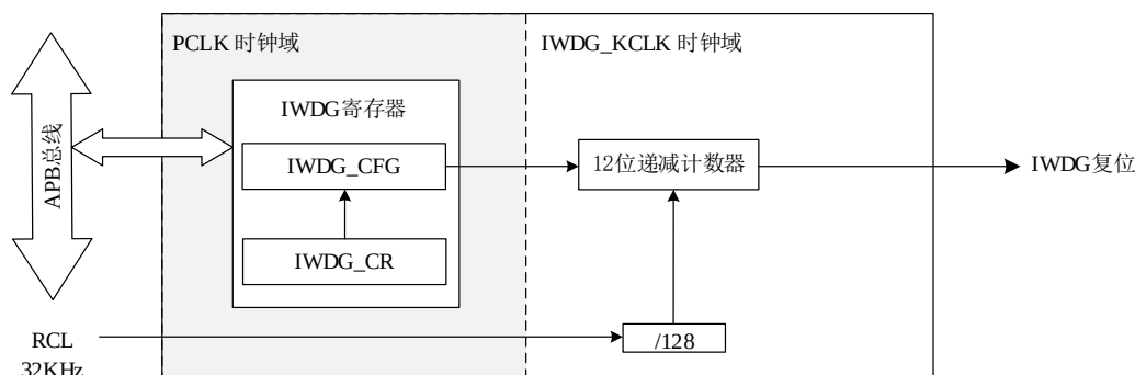
图 17-1 IWDG 框图
