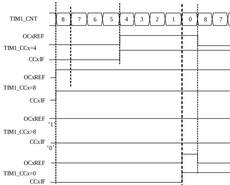
图 13-23 递减计数下的边沿对齐模式 PWM 波形（TIM1_ARR 寄存器为 8）
