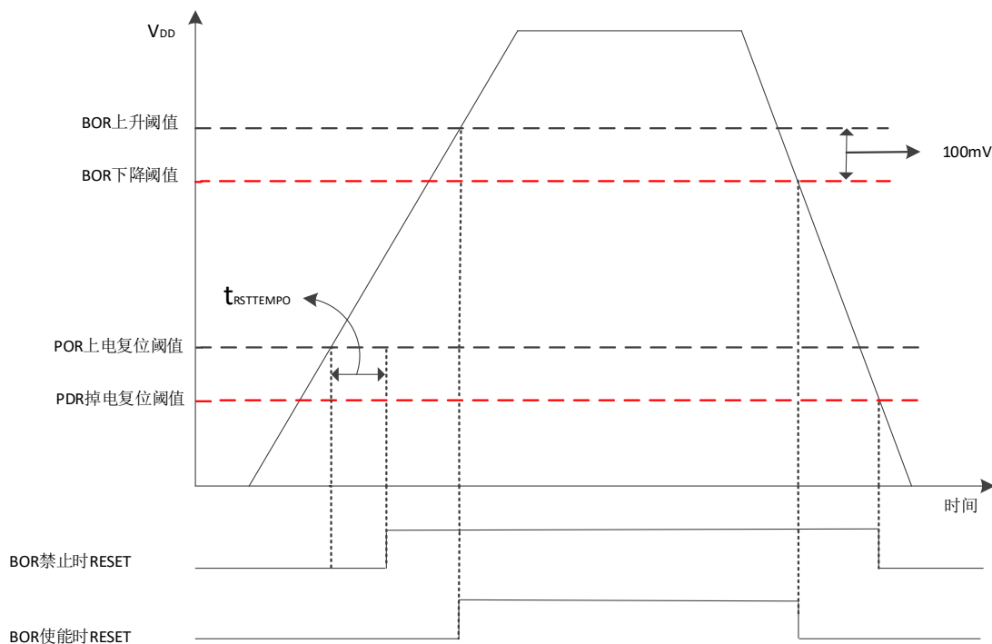
图 5-2 POR/PDR 和 BOR 阈值
