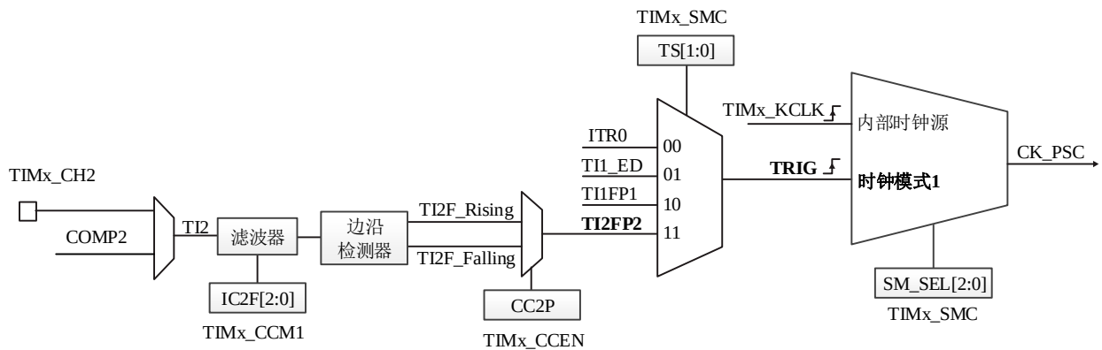
图 14-9 选择 TI2 作为时钟模式 1 触发输入的连接示例（上升沿计数）
