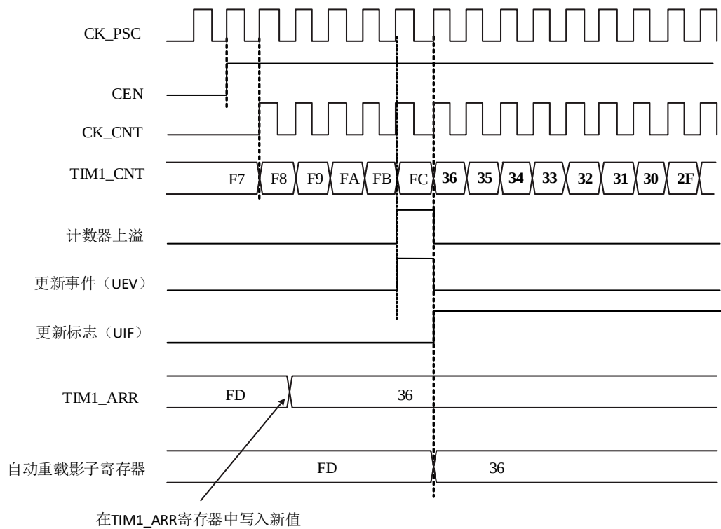
图 13-14 中心对齐模式下，产生上溢事件，ARPE=1 时的时序图
