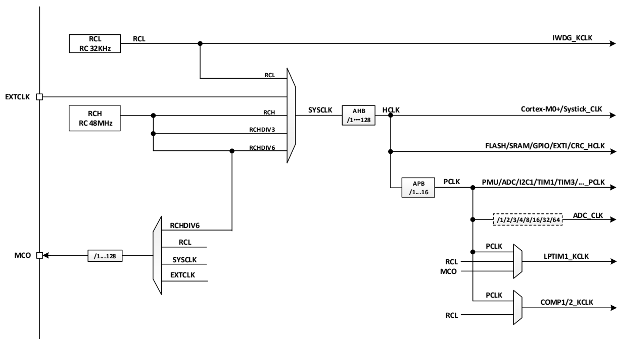
图 6-2 时钟树
