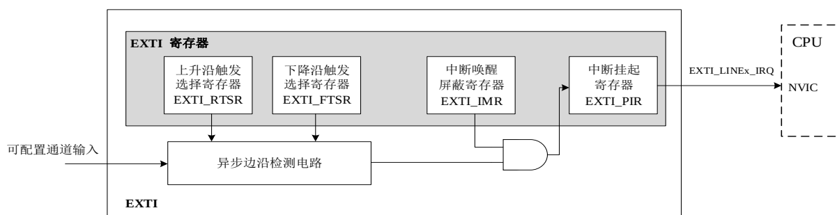
图 9-3 可配置通道的中断输出框图
