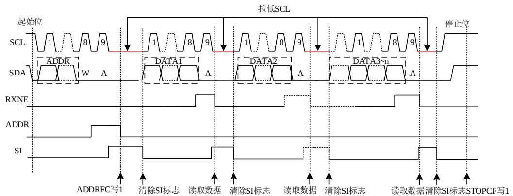
图 19-10 使能时钟低电平延长单字节控制接收数据
