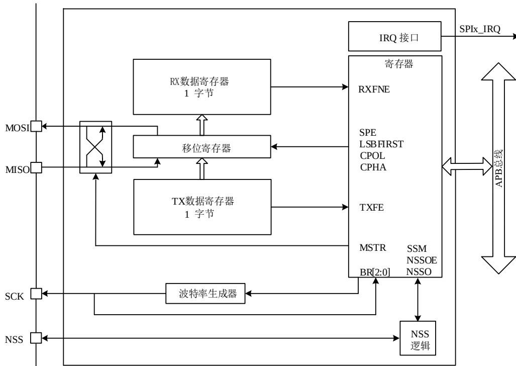
图 21-1 SPIx 框图 (x=1)
