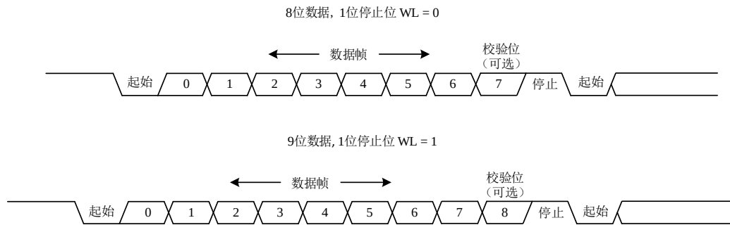
图 20-2 帧格式示意图
