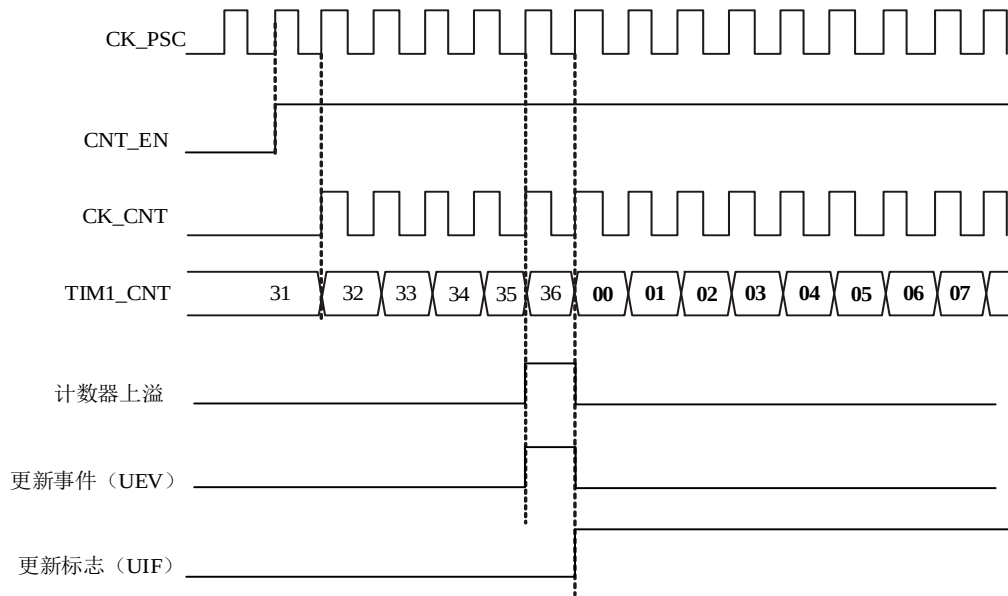
图 13-4 递增计数模式下配置预分频器为 1 分频上溢事件时序图
