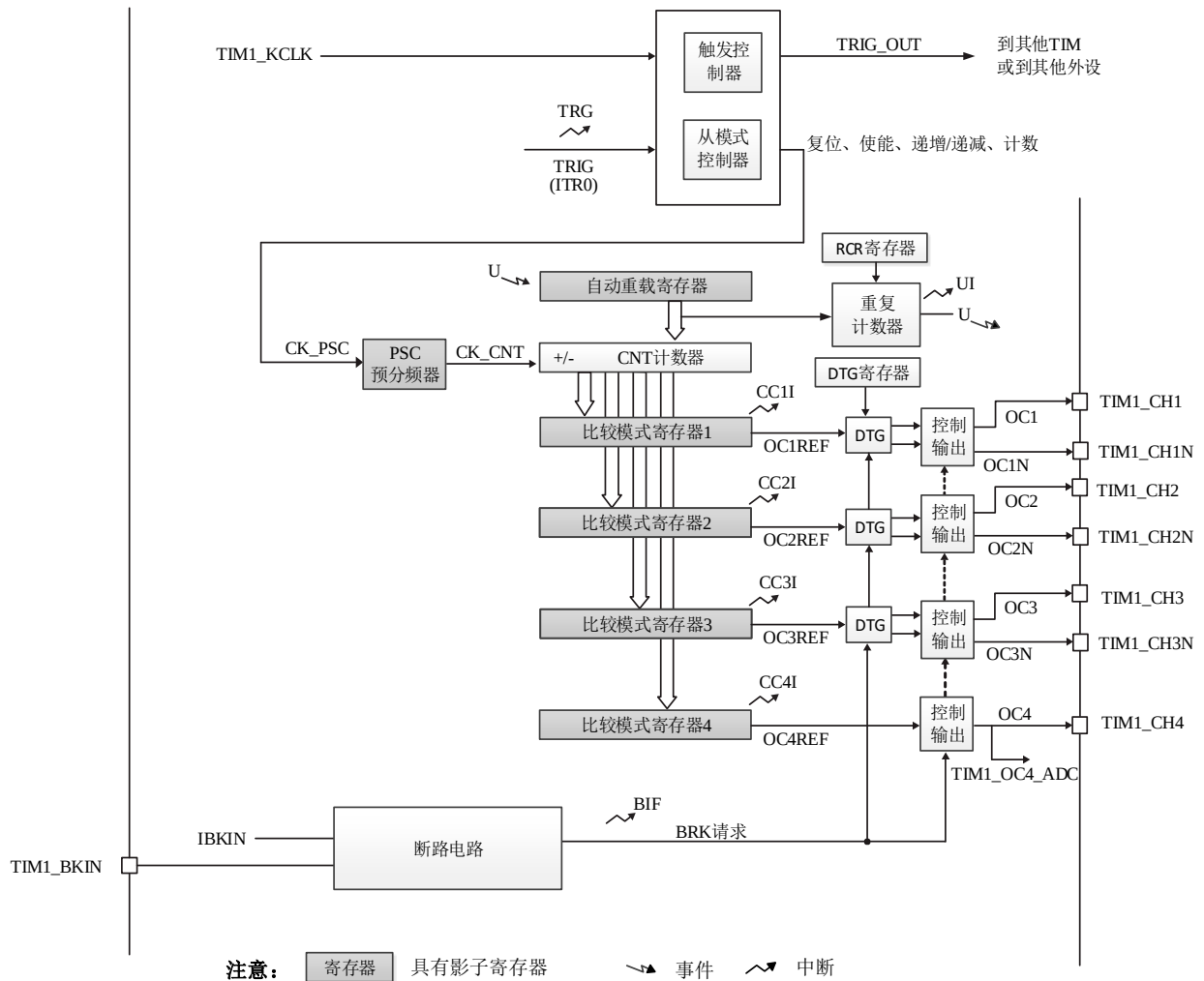
图 13-1 TIM1 框图
