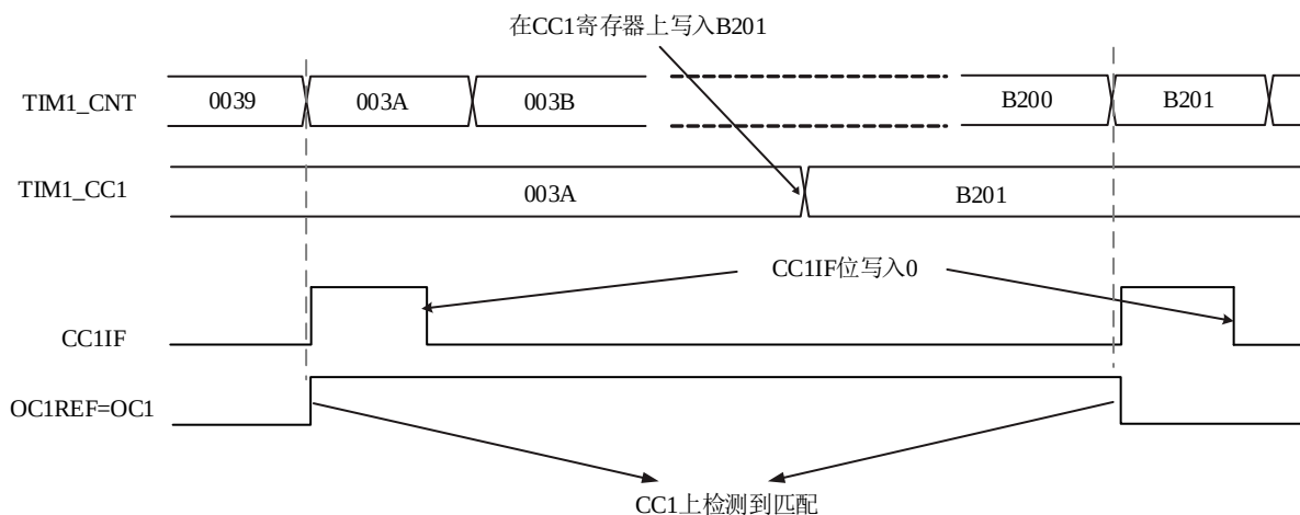
图 13-21 比较输出模式，翻转 OC1（OCxPE 位为 0）
