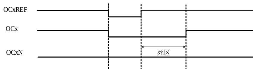
图 13-30 死区时间大于正脉冲宽度的死区波形
