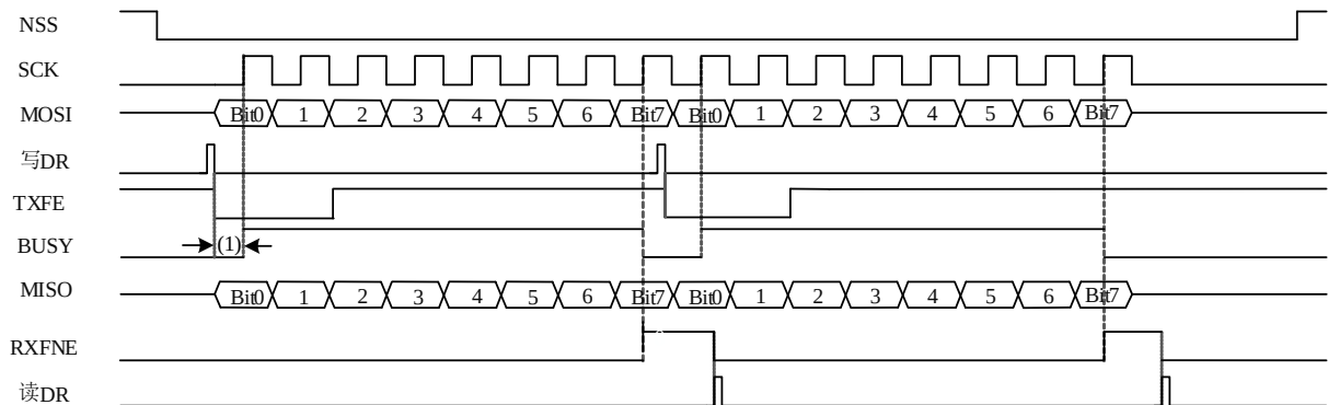
图 21-7 主模式通信时序
