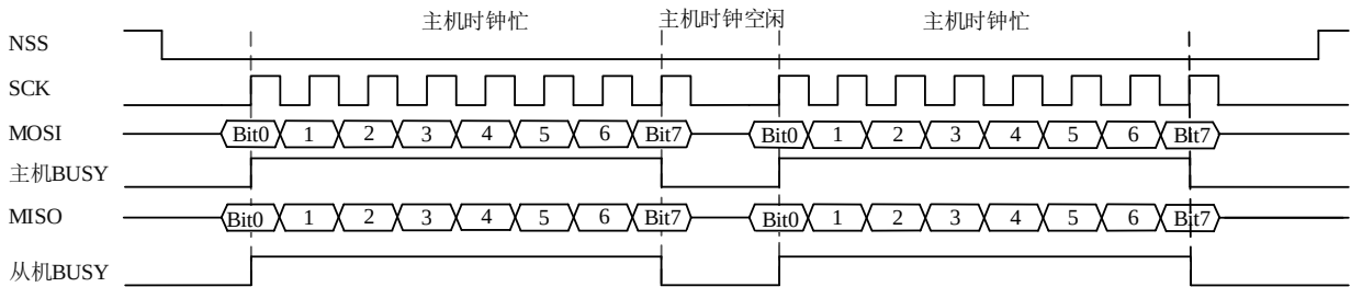
图 21-6 主从模式 BUSY 状态
