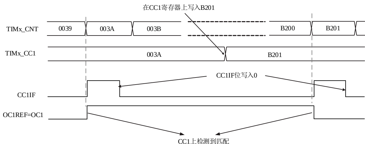
图 14-15 比较输出模式，翻转 OC1（OCxPE 位为 0）
