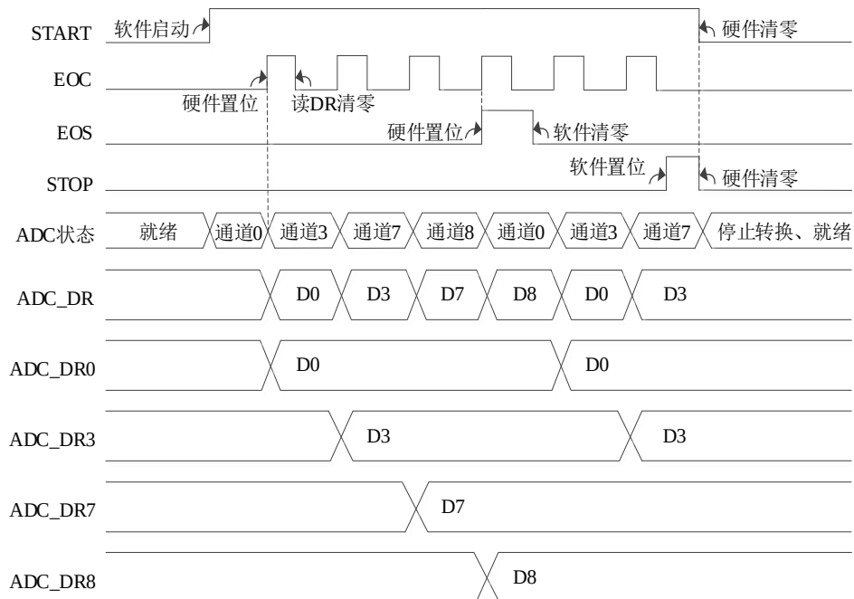
图 11-6 循环扫描转换模式，软件触发
