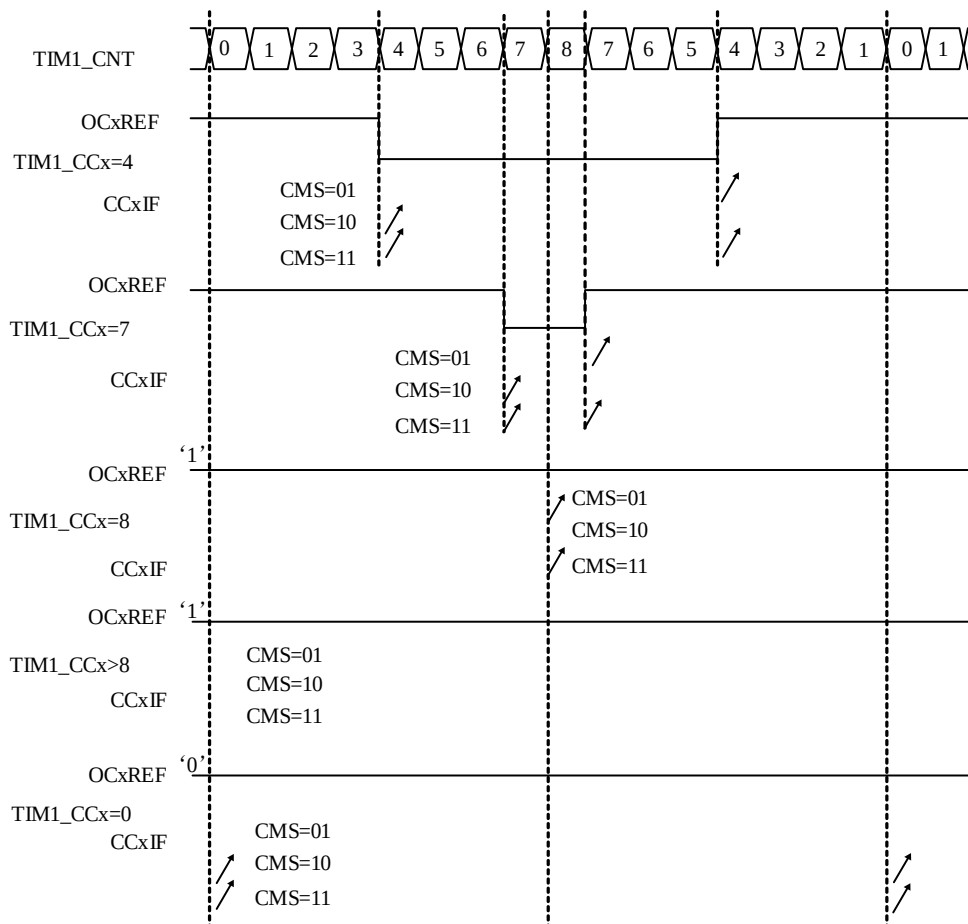
图 13-24 中心对齐模式 PWM 波形 (TIM1_ARR 寄存器为 8)
