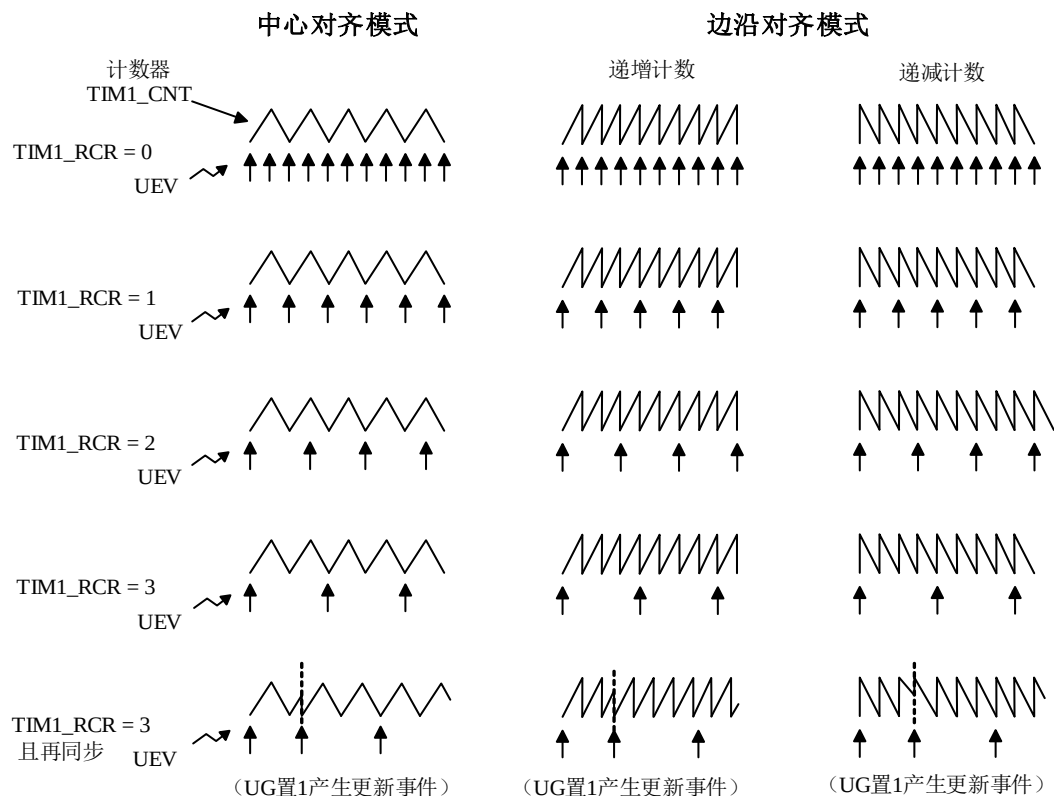
图 13-15 不同模式下设置不同 TIM1_RCR 寄存器值时的更新频率示例
