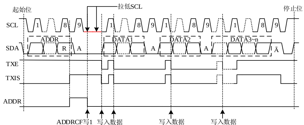
图 19-8 使能时钟低电平延长多字节控制发送数据
