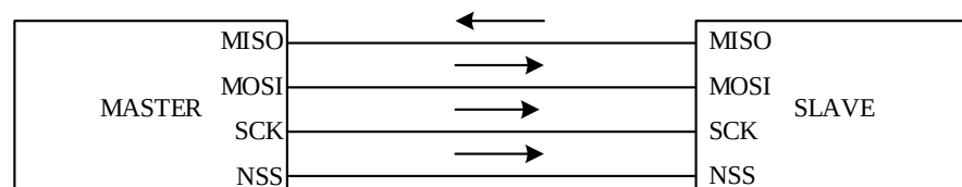
图 21-2 单主单从应用
