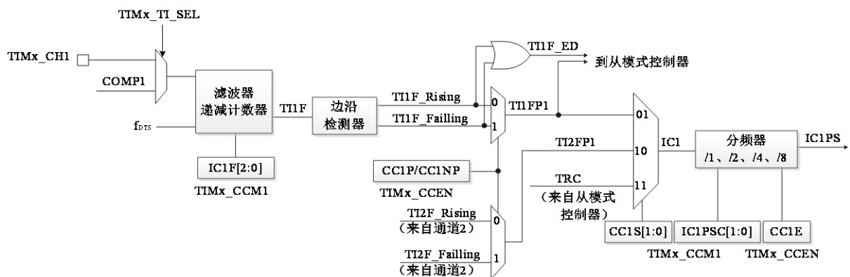
图 14-12 捕获/比较通道的输入连接图（通道 1）
