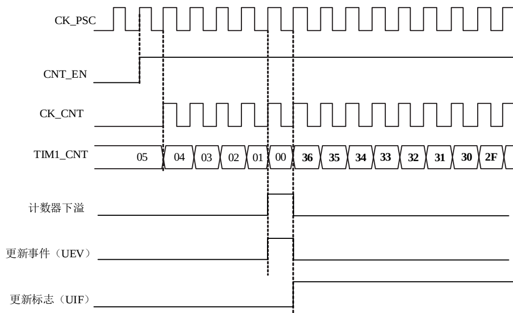
图 13-8 递减计数模式下配置预分频器为 1 分频下溢事件时序图
