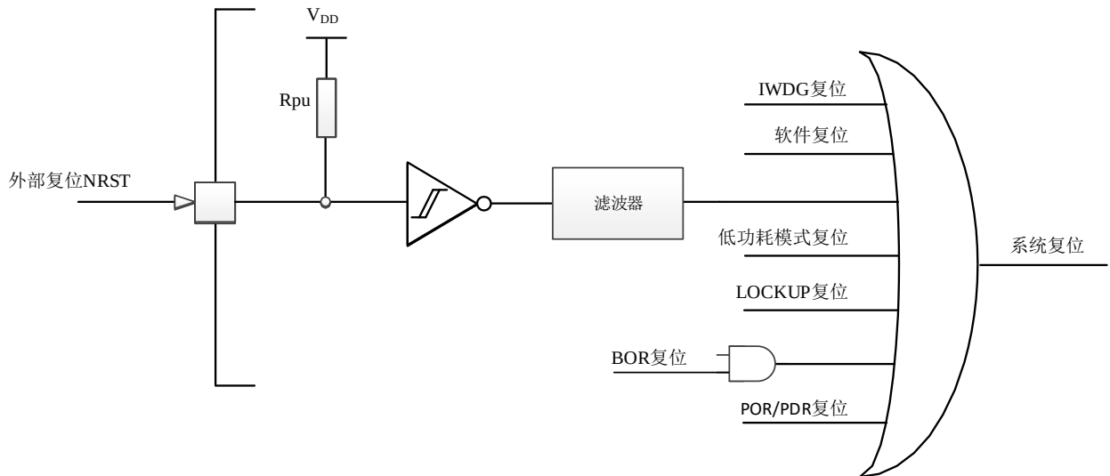
图 6-1 复位电路框图
