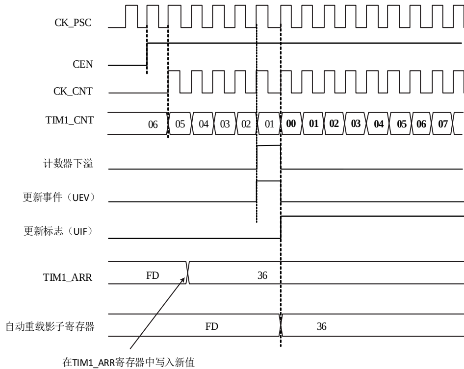
图 13-13 中心对齐模式下，产生下溢事件，ARPE=1 时的时序图
