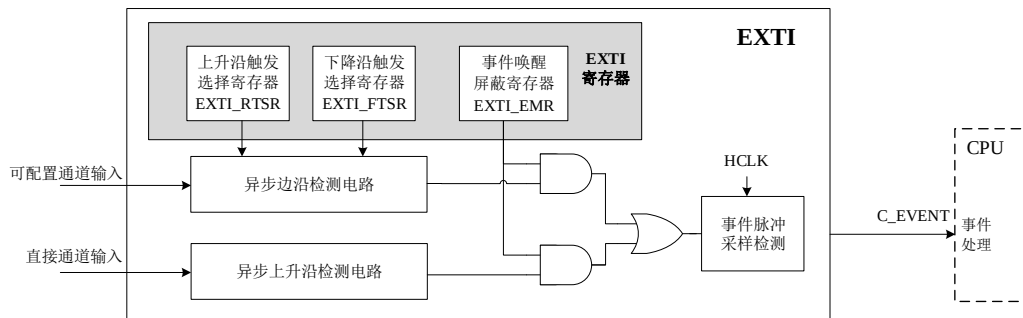
图 9-2 可配置通道&直接通道的事件输出框图
