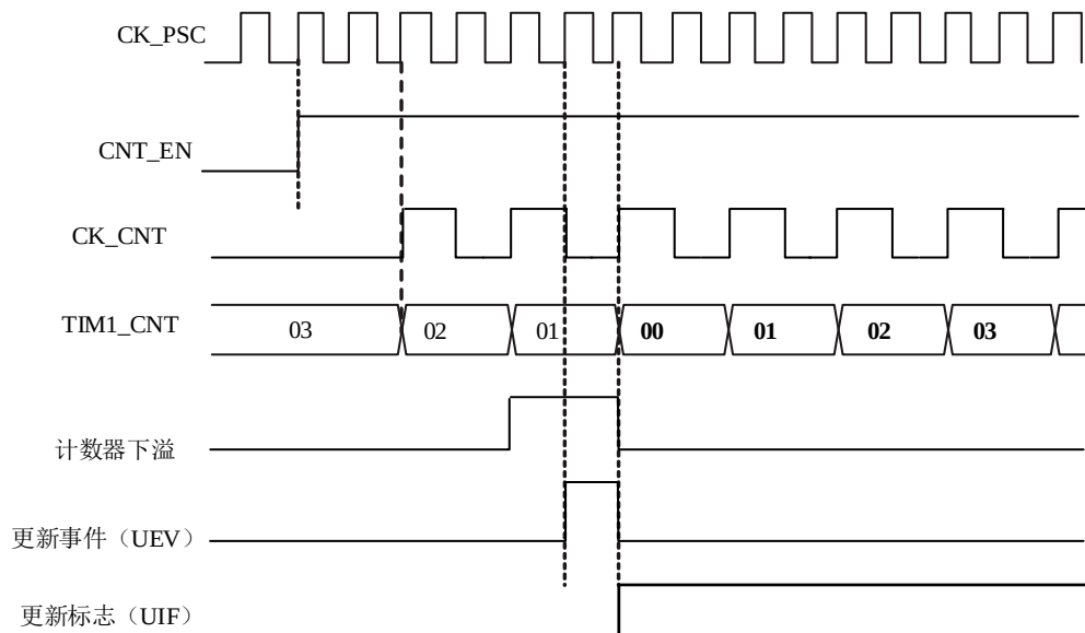
图 13-12 中心对齐模式下配置预分频器为 2 分频下溢事件时序图
