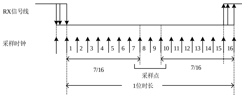
图 20-6 数据采样 (OBS=0)
