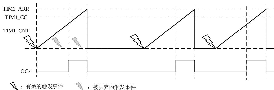
图 13-26 单脉冲输出波形
