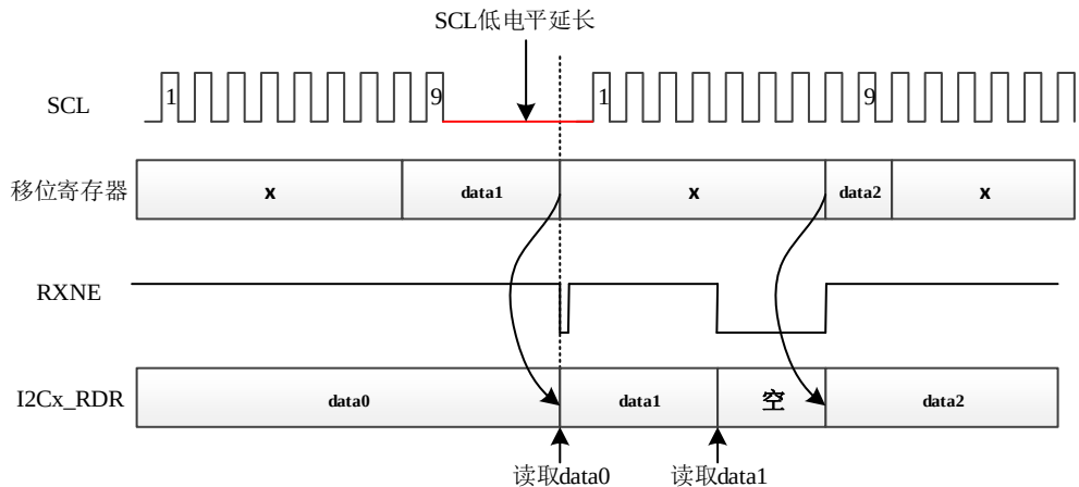
图 19-4 多字节控制数据接收
