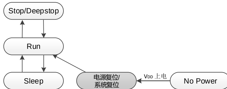
图 5-3 低功耗模式转换框图
