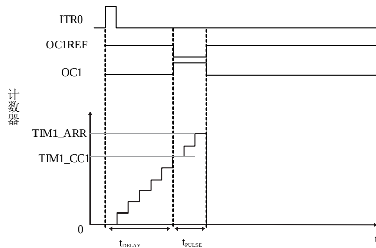
图 13-27 单脉冲模式示例
