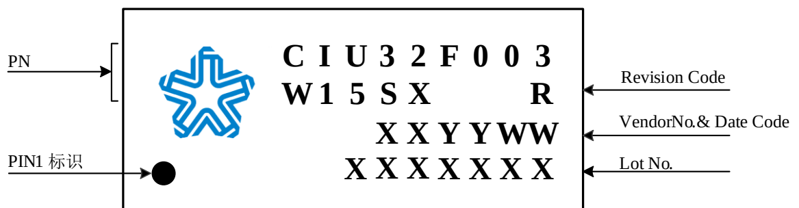
图 5-7 SOP16 type1 封装丝印信息说明
