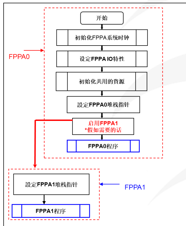
图 9：开机流程
