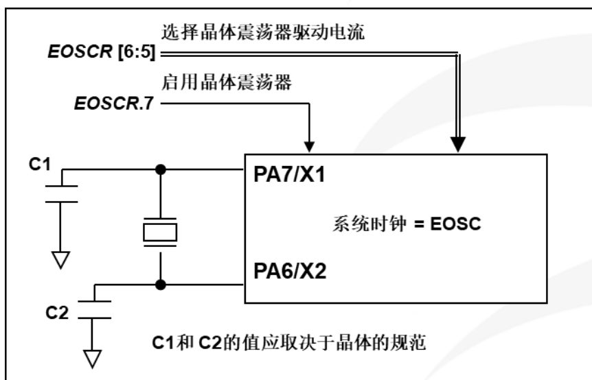
图 6: 外部晶体振荡器的的硬件连接
