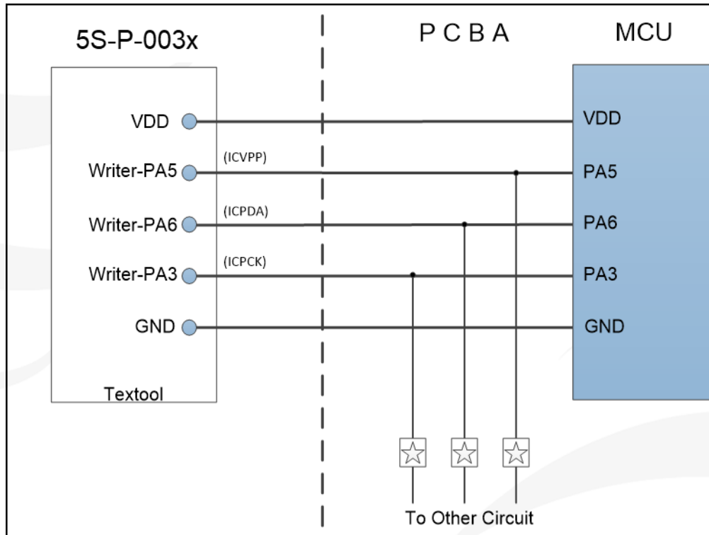
图 20：在板烧录接线示意图
